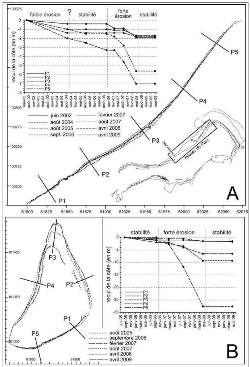
Fig. 12 – Cinématique du trait de côte des îles de Trielen et de Lez ar Chrizienn entre 2002 et 2009. Fig. 12 – Shoreline changes of Trielen and Lez ar Chrizienn Islands between 2002 and 2009.
