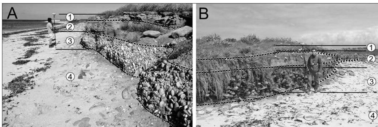
Fig. 5 – Plages éémiennees gélifées sur la côte nord de Trielen (A) et sur la côte sud de Lez ar Chrzienn (B). 1 : sol actuel ; 2 : dépôt périglaciaire (head) ; 3 : plage éémiennee gélifée ; 4 : plage actuelle.
