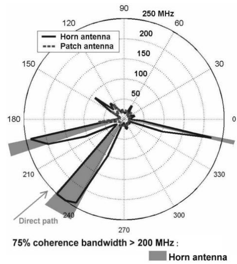
(a) CLE NLOS - B_{C_{75}} - RX07
