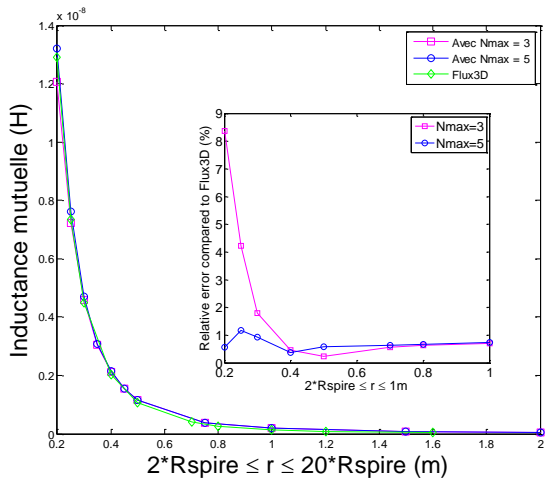
Fig.10 – Comparaison de l'inductance mutuelle entre deux boucles en fonction de la distance
