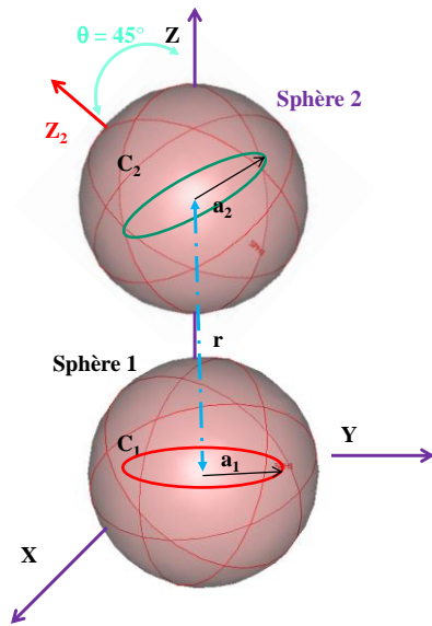
Fig.9 – Deux boucles de mêmes dimensions placées sur l'axe z où C_2 est à 45° du repère (x,y,z) .
