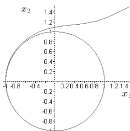
FIG. 4.2: Cercle unité : simulation de (4.14).
