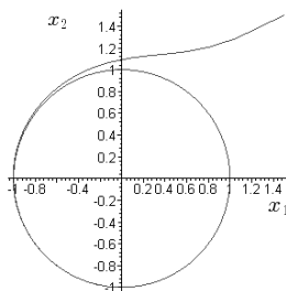
FIG. 4.5: Cercle unité : simulation de (4.36).
