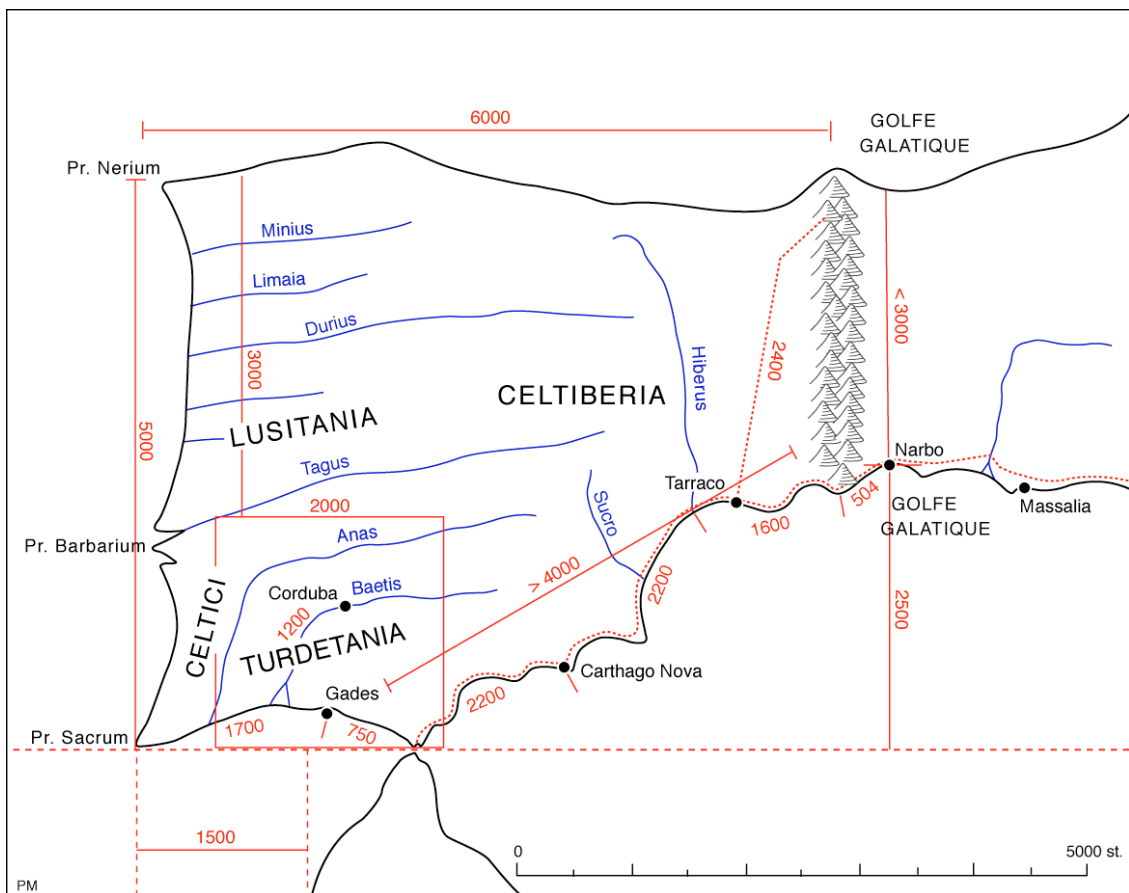
Fig. 7. Proposition de restitution des données cartographiques de Strabon.
