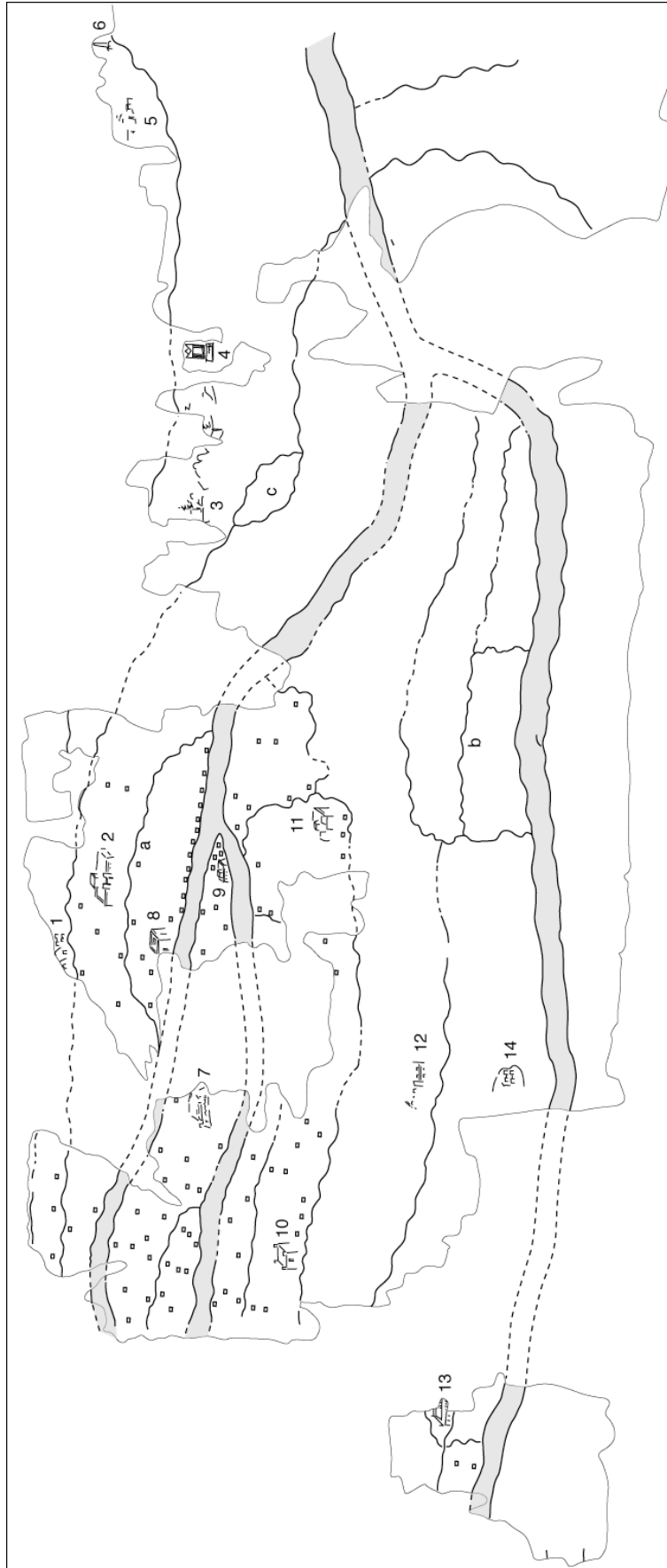
Fig. 1. La carte du papyrus d'après Gallazzi et al. , P. Artemid. (adapté). Les numéros des vignettes sont ceux des éditeurs ; les lettres a-b-c signalent des tracés qu'on peut interpréter comme des canaux.
