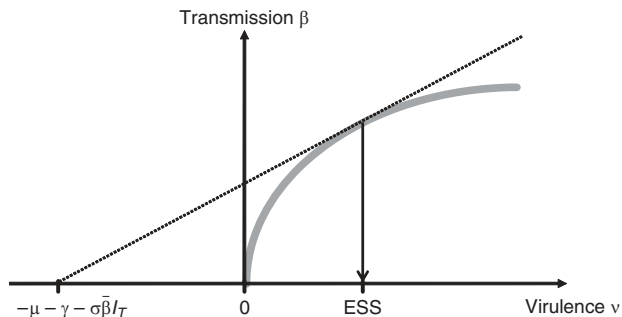
Figure 40 Construction géométrique permettant de retrouver les conséquences qualitatives de différents paramètres du modèle sur la stratégie évolutivement stable de virulence du parasite. Étant donné une fonction décrivant le compromis (courbe grise) entre transmission et virulence, la stratégie évolutivement stable de virulence est obtenue après avoir trouvé la droite (en pointillée) tangente à cette fonction et qui passe par le point \{0, -\mu - \gamma - \sigma \bar{I}_T\} . L'abscisse du point de tangence donne la valeur de la virulence qui satisfait la condition (8), et correspond donc à la stratégie de virulence évolutivement stable (ESS).
