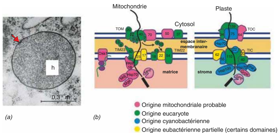
Figure 37 Deux aspects de la coévolution dans le cas des organites endosymbiotiques. (a) Mitochondrie modifiée (ou hydrogénomosome) d'eucaryote anaérobie Trichomonas foetus , limitée par deux membranes (flèche) mais ne possédant plus de génome (cliché Marlene Benchimol, Santa Ursula University). (b) Origines des translocases mitochondriales et plastidiales, qui transfèrent les protéines synthétisées dans le cytosol vers ces organites. Plus de 25 protéines forment les complexes TOM (translocase de la membrane externe mitochondriale) et les deux
