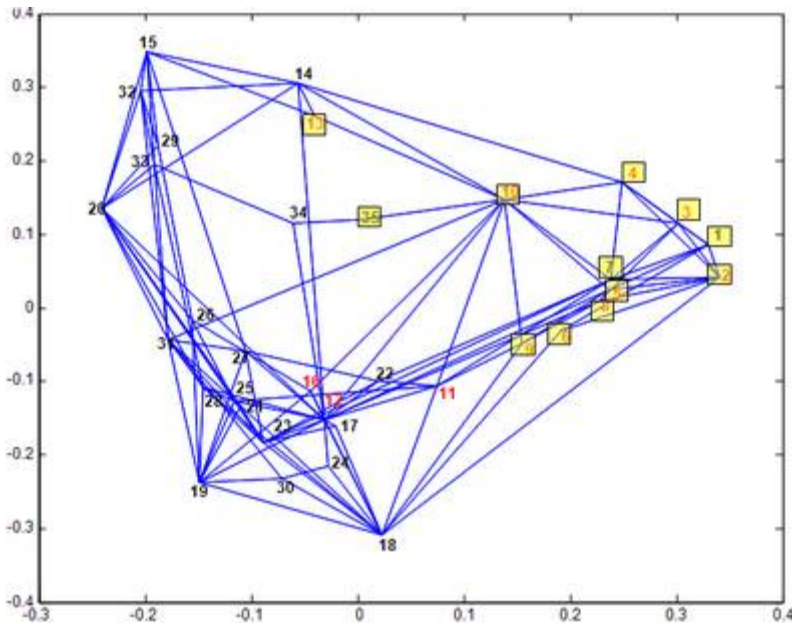
Figure 10. L'espace intrinsèque ( U_2, U_3 ) du graphe des liens entre hommes politiques mexicains. En rouge les militaires, en surligné jaune notre partition optimale.
