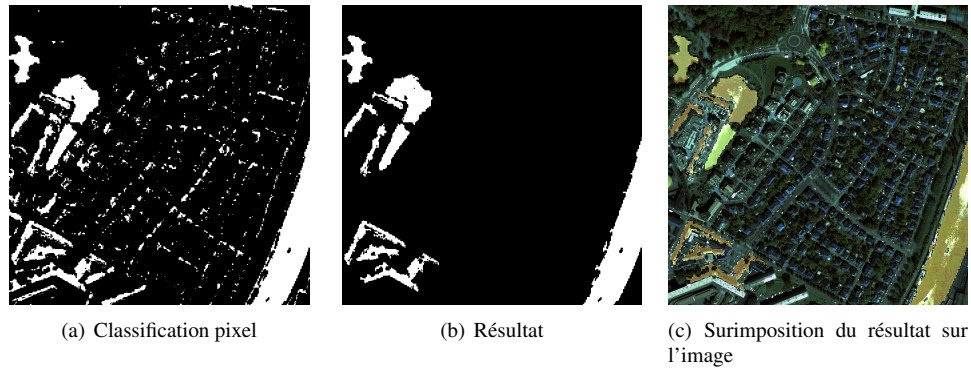
FIG. 7 – Application du détecteur pour le concept eau.
