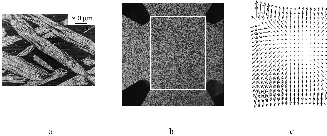
FIG. 1 – a -microstructure du composite. b -Éprouvette et région d'étude (rectangle blanc). c -Champ de déplacement mesuré par corrélation d'images pour un niveau d'effort (11 kN) proche de la rupture (11.1 kN).
