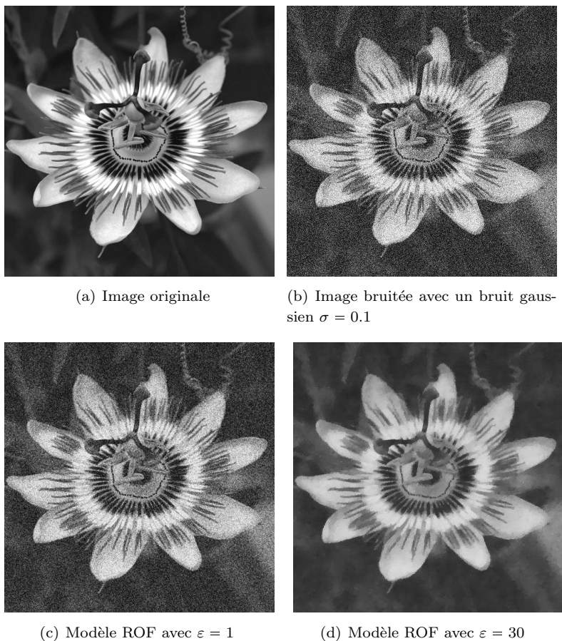
FIGURE 26. Filtrage ROF : sensibilité au paramètre \varepsilon
