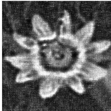
(d) Itération 20
