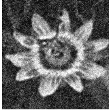
(b) Itération 5
