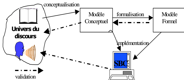
Fig. 1 Cycle de vie d'un SBC
