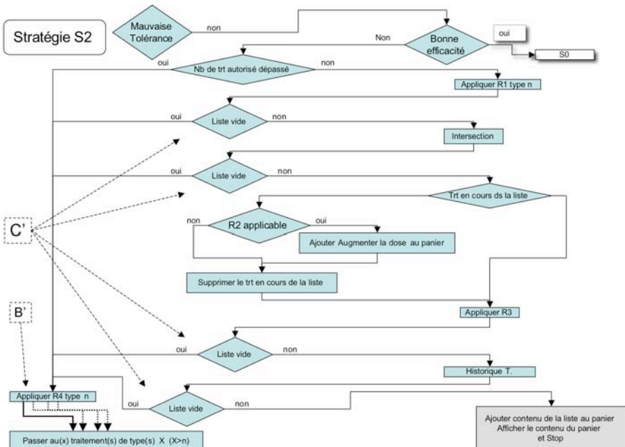
Fig. 2 – Organigramme de séquences d'exécution au cours de la stratégie S2. En haut est présentée la 1 ère version et au-dessous la version enrichie et explicitée.
