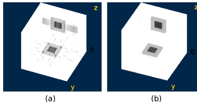
fig.2 Phantoms reconstruits avec 16 projections en Feldkamp (a) et avec notre méthode (b)
