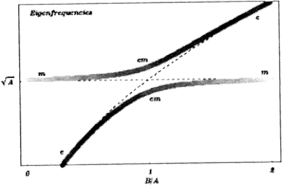
Fig. 6. Veering of eigenfrequencies
