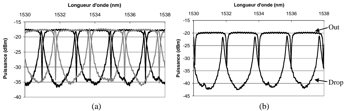
Fig. 2 : Spectres mesurées sur les sorties "Out" et "Drop" de micro-résonateurs de rayon de courbure R = 120 μm. (a) Espacement entre guide et anneau : 0,7 μm. (b) espacement entre guide et anneau : 0,8 μm.
