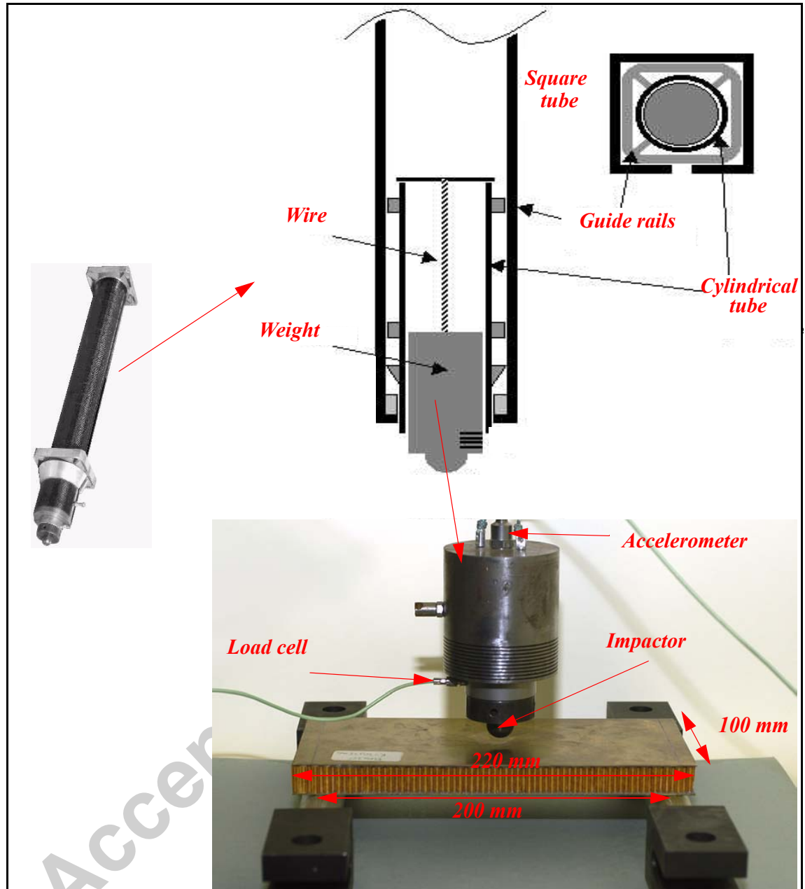
Figure N° 19 : Load drop test rig.
