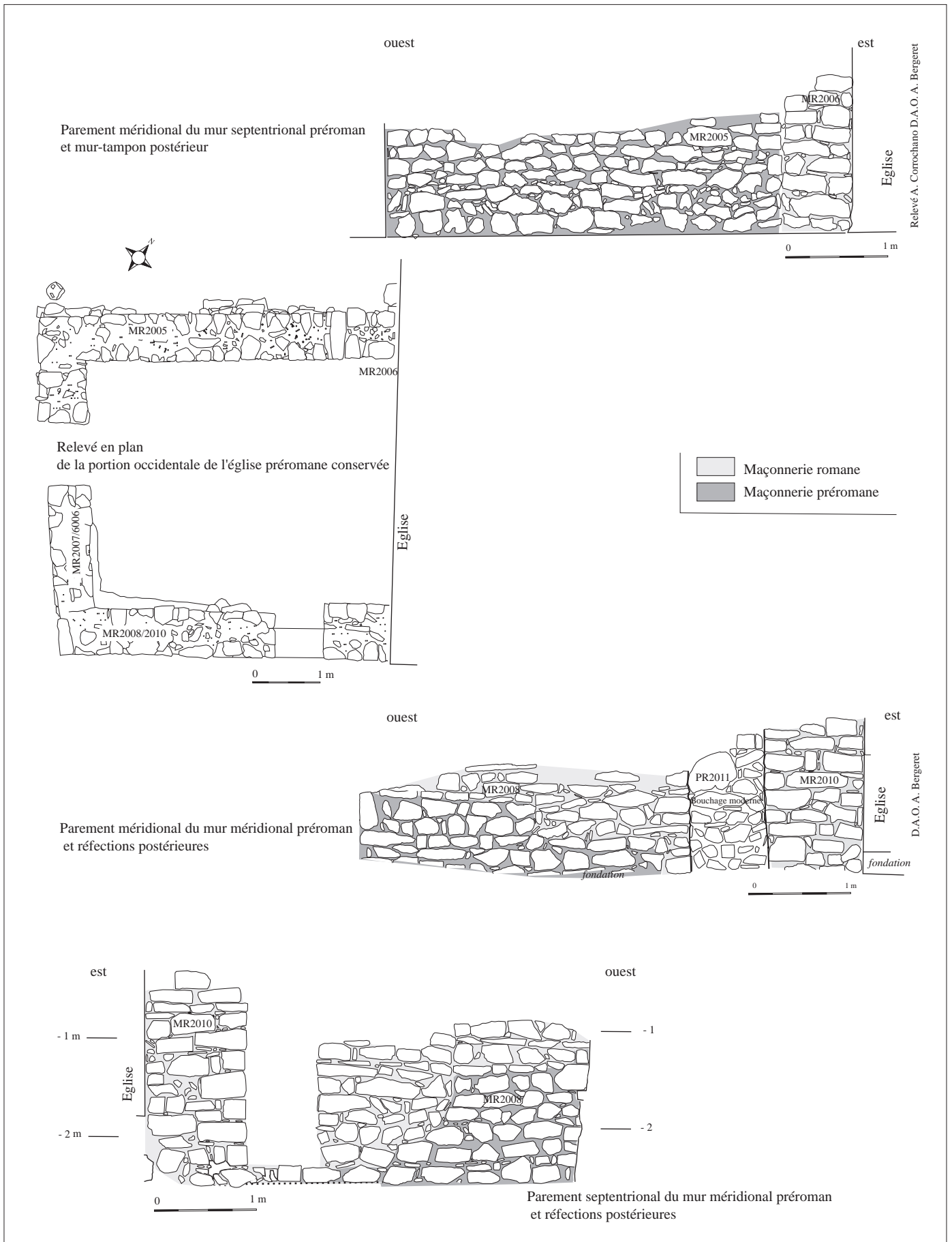
Fig. 6 - Vestiges de l'église préromane, relevé en plan et en élévation des maçonneries.
