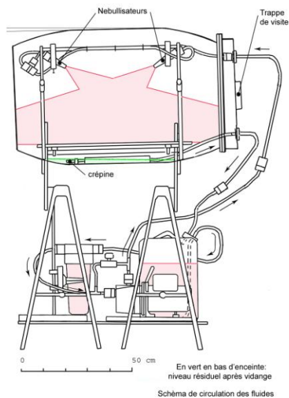
Encart 3 : machine à former et à rincer, pression du fluide circulant 3 bars: en mode dit de «fixation» la détente via les nébulisateurs assure la vaporisation du formol en vase clos
