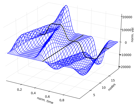
(d) velocity
