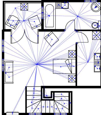
Figure 5. Visualisation du graphe d'adjacence de région extrait sur un plan de la base floorplans
