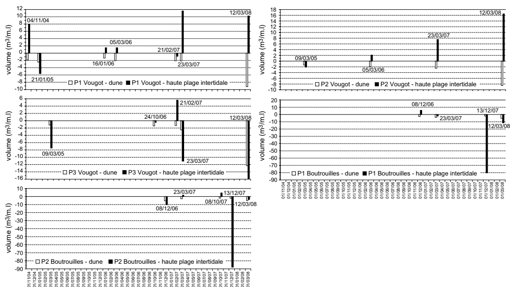
Figure 14 : Bilans sédimentaires (en \text{m}^3/\text{m.l.} ) de la dune et de la haute plage intertidale des plages du Vougot et de Boutrouilles pour les phases érosives majeures enregistrées depuis 2004
