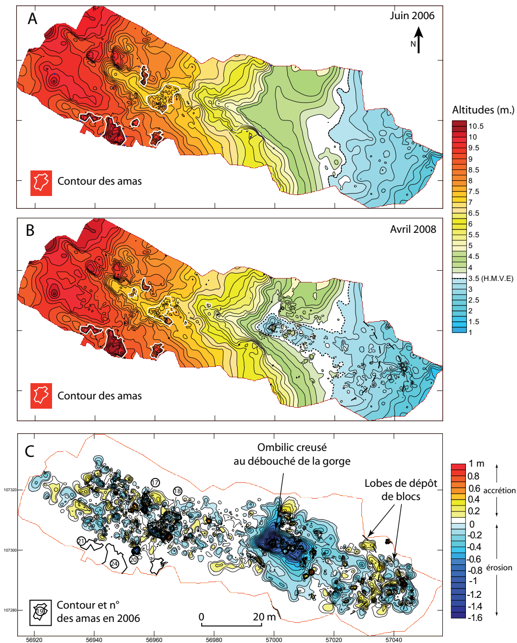
Figure 5 : Modifications de la topo-morphologie de la gorge et de ses abords, au centre de l'île de Banneg, lors de la tempête du 10 mars 2008
