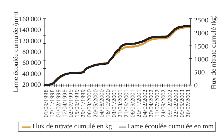
▼ Figure 1 – lame écoulée et flux de nitrate : cumuls des valeurs journalières mesurées du 1 er septembre 1998 au 31 août 2003 à l'exutoire du bassin versant de la Fontaine du Theil à Saint-Léger.
