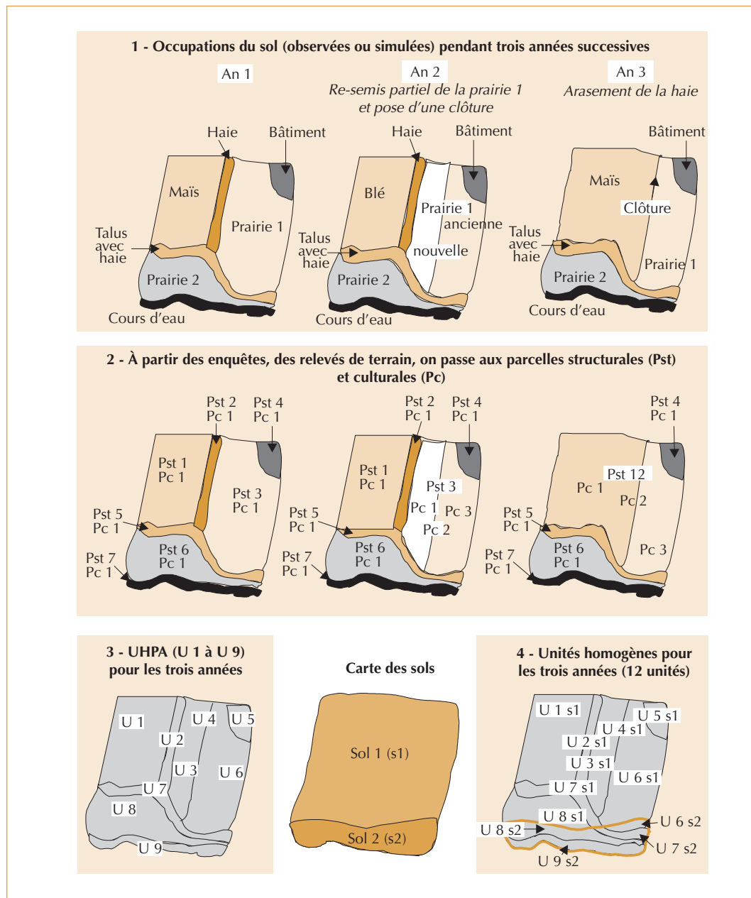
► Figure 4 – Principes de discrétisation horizontale de l'espace utilisés par le modèle BMP1top.
