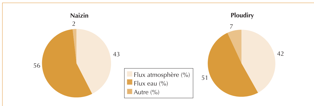
◀ Figure 6 – Répartition de l'excédent du bilan azoté entre les flux dans l'eau et dans l'atmosphère pour les bassins versants de Naizin et Ploudiry en % de l'excédent du bilan de l'azote.
