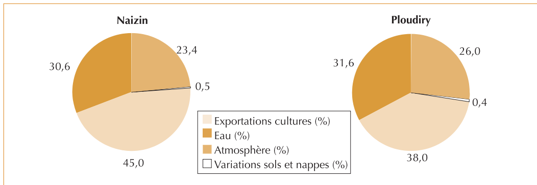
◀ Figure 5 – Répartition des apports azotés entre les exportations par les cultures, les flux dans l'eau et l'atmosphère sur les bassins versants de Naizin et Ploudiry pour le scénario BPA0.
