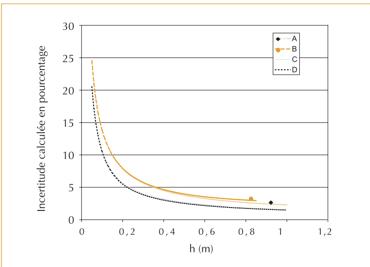
▼ Figure 12 – Calcul théorique des incertitudes sur la surface de la section mouillée pour quatre stations. A, B, C et D correspondent aux stations définies dans la figure 9 (p. 31).
