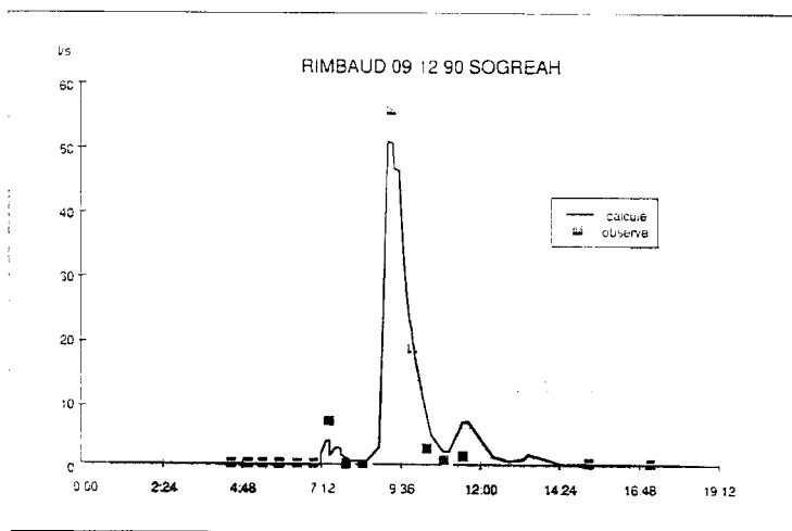
Figure 7. – Rimbaud, crue du 9 décembre 1990 ; sédimentogramme transitité. Comparaison calculé/observé
