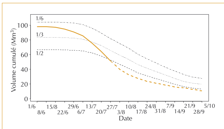
▲ Figure 6 – Courbes de défaillances (traits pointillés fins) et courbe de déstockage (trait brun continu et pointillé gras) pour le système Neste en 2003. Les courbes de défaillances représentent les volumes minima qu'il faut avoir en stock pour satisfaire la demande avec un risque de défaillance donné (par exemple 1 année sur 6, sur 3 ou sur 2). Ces courbes sont établies en fonction des ressources disponibles. La courbe de déstockage représentée ici est une courbe observée jusqu'au 29 juillet (trait continu brun), puis simulée (trait pointillé). Les simulations intègrent les estimations de prélèvements d'irrigations faites avec ADEAUMIS.
