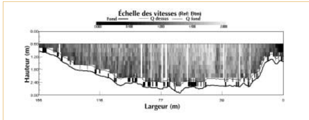
► Figure 4 – Répartition des vitesses sur le profil n° 3 de Lamagistère, campagne de mai 2003 (vitesses les plus faibles représentées en sombre et les plus rapides en clair).
