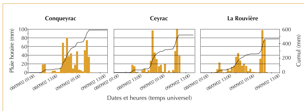
◀ Figure 4 – Pluviogrammes au droit des barrages de Conqueyrac (relevé manuel), Ceyrac et La Rouvière (relevés automatiques) – Source : syndicat mixte interdépartemental d'aménagement et de mise en valeur du Vidourle et de ses affluents.
