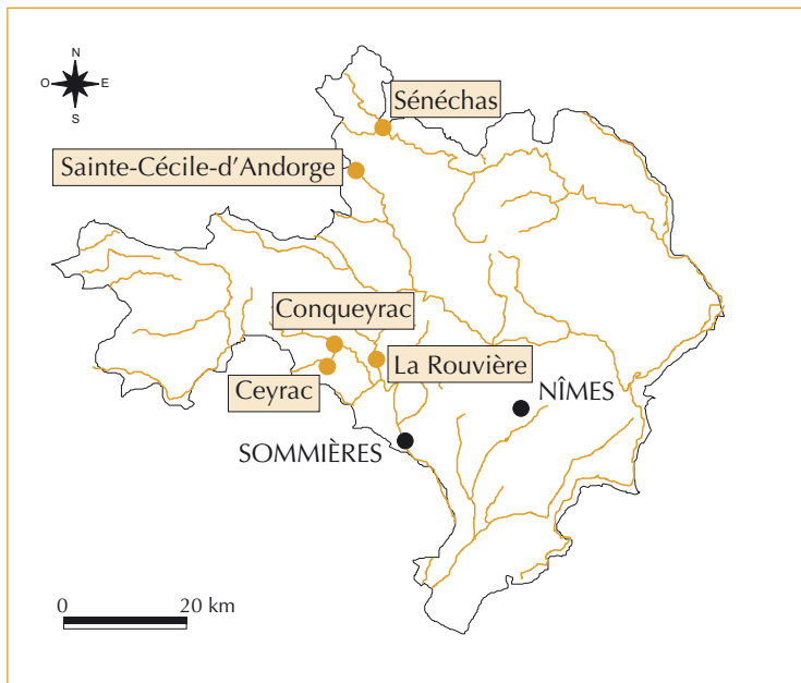
▼ Figure 2 – Localisation des barrages écrêteurs de crues du département du Gard.
