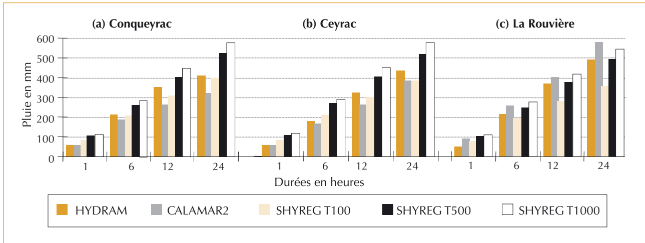
▲ Figure 8 – Confrontation des pluies maximales de bassin en 1, 6, 12 et 24 h avec les quantiles rares de la pluie de bassin.
