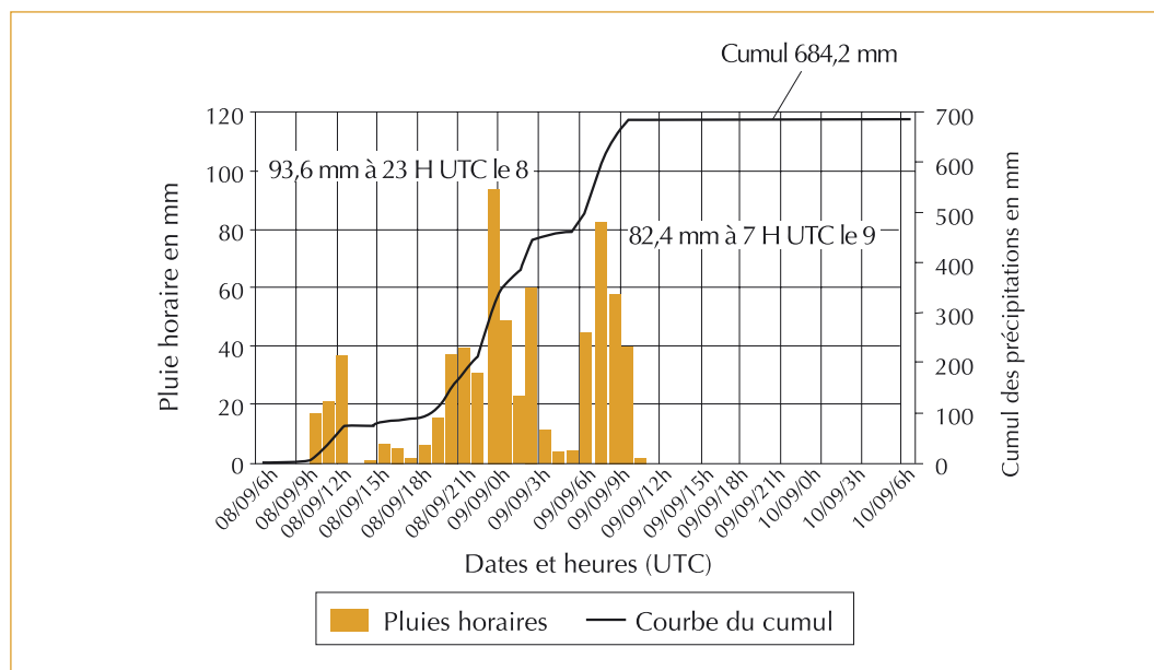
◀ Figure 1 – Hyéto-gramme du pluviographe de Cardet du 08/09/2002 à 6 h au 10/09/2002 à 6 h TU (temps universel) – Source : Météo-France.
