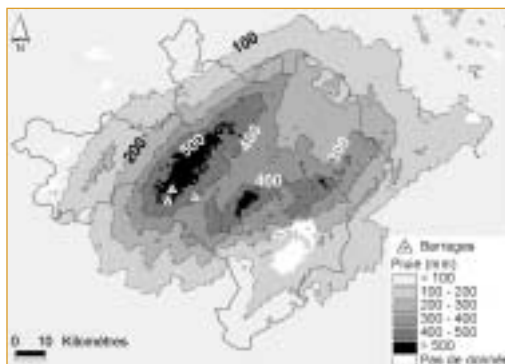
◀ Figure 5 – Pluies radar Météo-France en 48 h à partir de 00 h 00 TU le 08/09/02.
