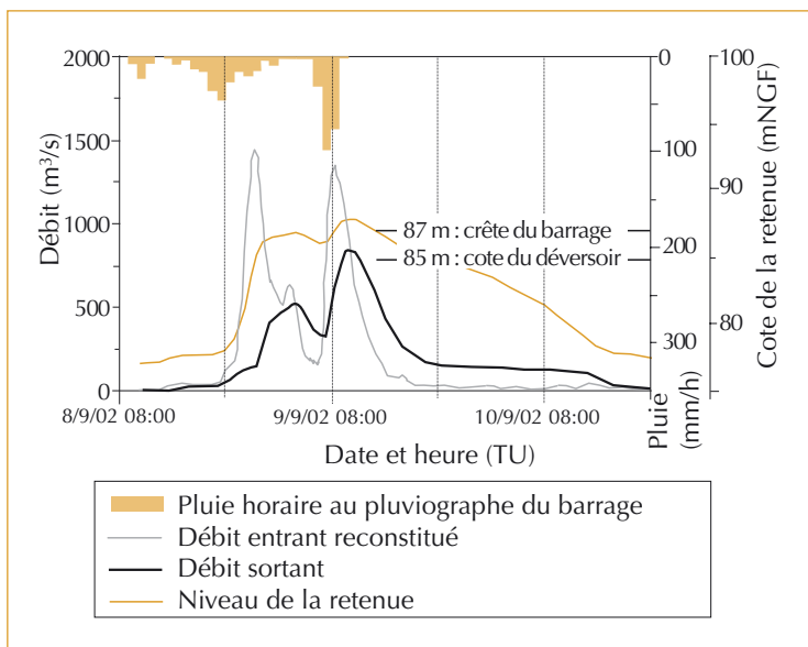
▼ Figure 10 – Hydrogrammes au barrage de la Rouvière.
