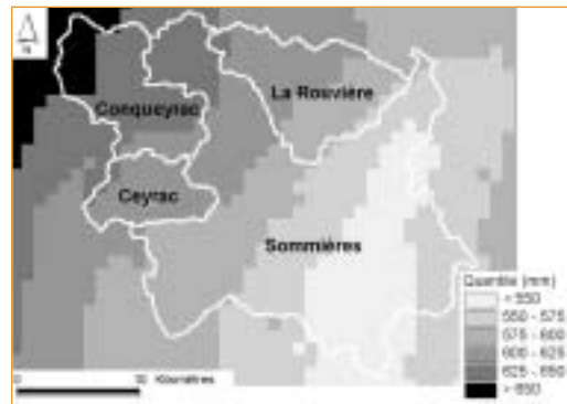
► Figure 6 – Estimations SHYREG de la pluie millénaire maximale en 24 h.
