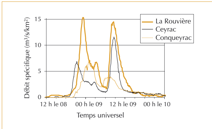
▲ Figure 9 – Débit spécifiques reconstitués à l'entrée des retenues des barrages écrêteurs du Vidourle.
