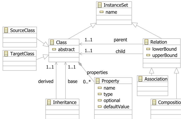
Figure 2 – Méta-modèle source et cible
