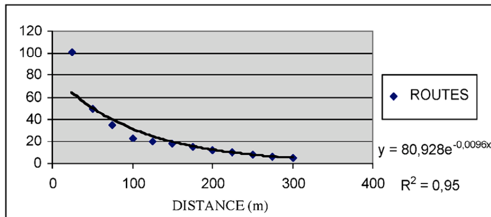
Fig. 5. Relation entre le nombre de départs de feu (ordonnée) et la distance à la route (par pas de 25 m) dans les Alpes-Maritimes de 1991 à 2003. Source : J.G. ROBIN, 2006.
