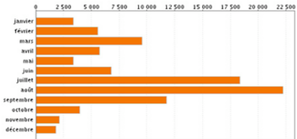
Figure 2. Nombre mensuel total d'incendies de forêts ayant affecté les 15 départements du Sud-Est de la France de 1973 à 2007. Source : Prométhée.
