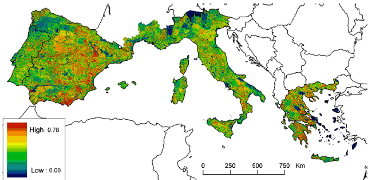
Figure 8. Probabilité d'éclosion à partir de la teneur en humidité des plantes, le 10 août 2004. Source Eufirelab.
