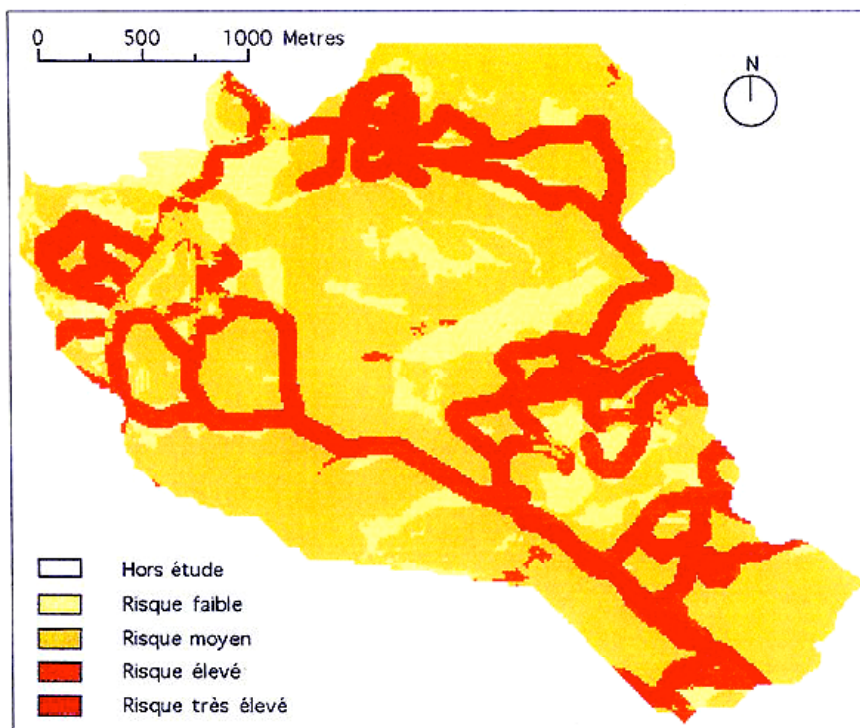
Figure 6. Spatialisation de l'indice d'écllosion de CHUVIECO (hors facteurs météorologiques) sur la commune de Valbonne (Alpes-Maritimes). Source : R. BLANCHI, 1996.
