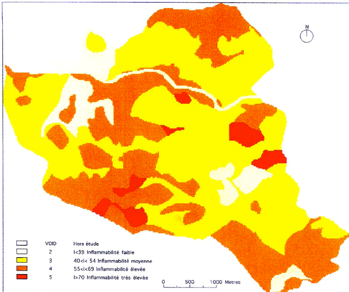
Figure 3. Carte de l'indice d'inflammabilité (hors facteurs météorologiques) sur la commune de Valbonne (06). Méthode Alexandrian (1982). Source : R. BLANCHI, 1996.
