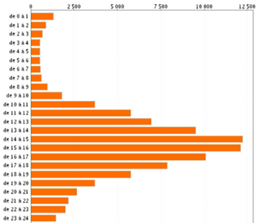
Figure 7. Heures de départ des feux dans le Sud-Est de la France, de 1973 à 2007. Source : Prométhée.
