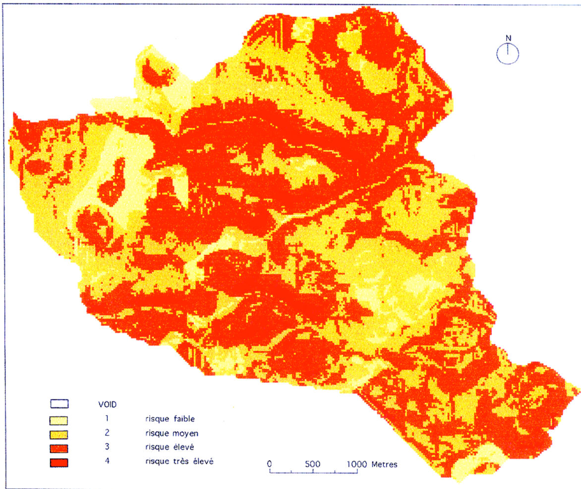
Figure 4. Carte du risque de propagation (hors facteurs météorologiques) sur la commune de Valbonne (06). Méthode Chuvieco. Source : R. BLANCHI, 1996.
