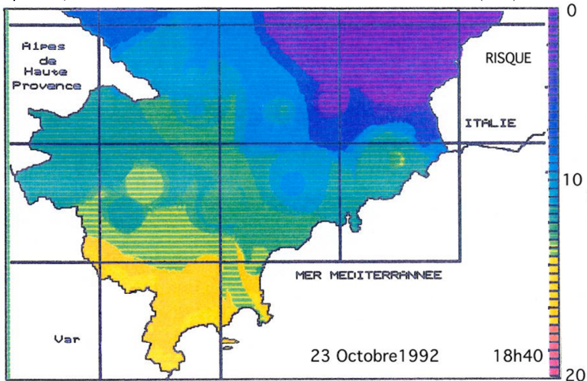
Figure 9 Carte du risque météo d'incendie de forêt (indice Carrega I85/90) calculé à fine échelle spatiale (pixel 200m) utilisé opérationnellement de 1990 à 2000 par le Service de Défense Incendie et de Secours (SDIS) des Alpes-Maritimes (exemple du 23 octobre à 18h40).
