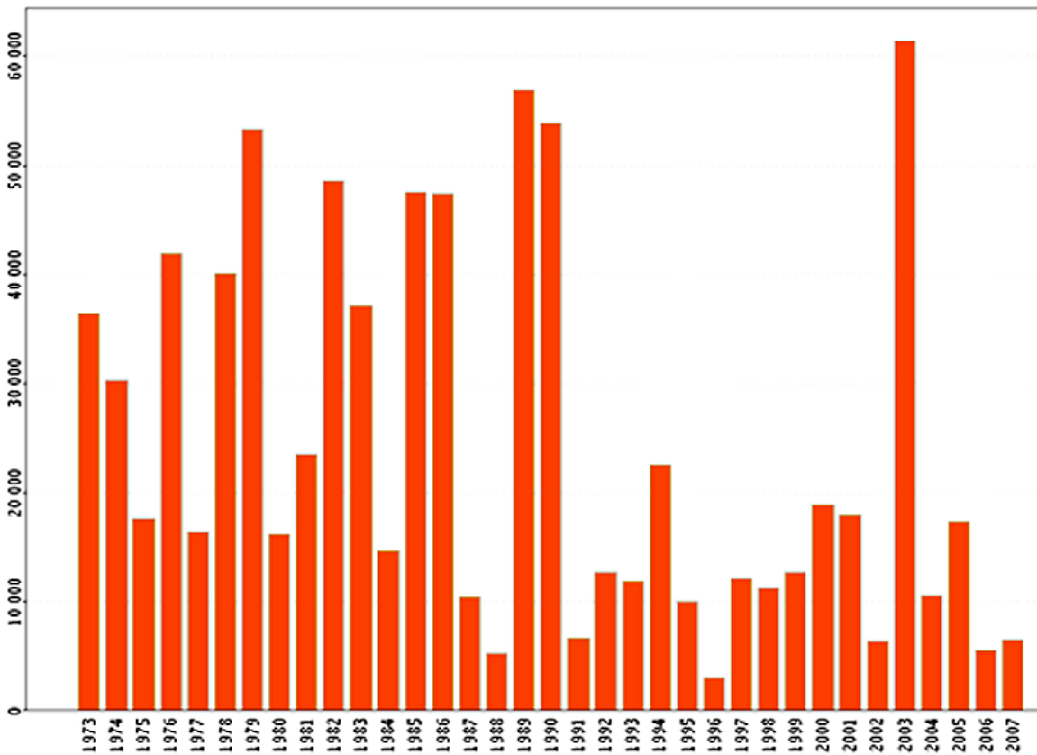
Figure 1. Nombre total annuel des incendies de forêts ayant affecté les 15 départements du Sud-Est de la France (proches de la Méditerranée) de 1973 à 2007. Source : Prométhée.
