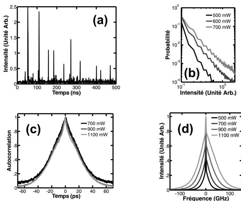
FIG. 2 : Signal amplifié (a) Visualisation à l'oscilloscope (b) Statistique correspondante (c) Signal d'autocorrélation pour différentes puissance de pompe (d) Evolution du spectre pour les puissances indiquées
