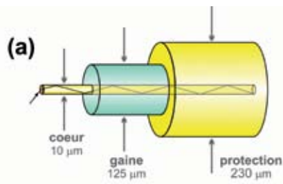
Fig. 3 [a] Principe d'une fibre optique : la lumière est transportée dans le cœur de la fibre dont le diamètre est de quelques millièmes de millimètres seulement.
