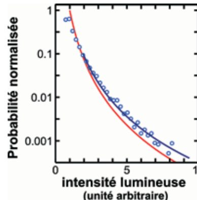
Fig. 10 Distribution de probabilité de l'intensité maximale des impulsions après amplification. Les intensités lumineuses et leur probabilité sont normalisées par rapport à la valeur moyenne. Les résultats expérimentaux (cercles) suivent une courbe décroissante exponentielle (sur une échelle logarithmique) caractéristique des phénomènes rares. Nos observations expérimentales sont comparées avec les prédictions numériques (courbe rouge).
