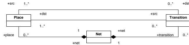
(a) Petri Net MM1 (version 0)
