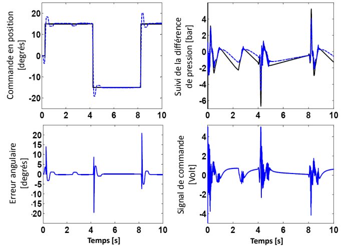
Fig. 5. Réponse à un signal carré (vérin sans tige)
