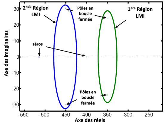
Fig. 6. Pôles et zéros : région LMI de type cercle et emplacement des pôles en boucle fermée
