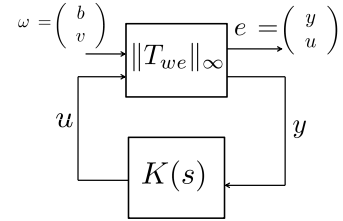
Fig. 3. Schéma de commande et notations
