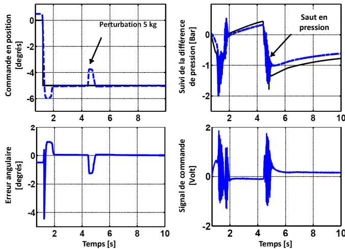
Fig. 8. Test de robustesse avec une masse de 5\text{kg} : un saut dans la différence de pression est observé lors de l'ajout de la masse. La stabilité et les performances du système sont préservées.
