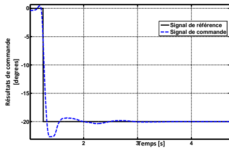
Fig. 7. Réponse indicielle pour un gain élevé (pôles rapides)
