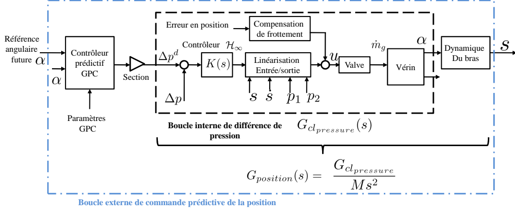
Fig. 4. Stratégie de commande en cascade position/pression pour les vérins pneumatiques. Une boucle interne consiste en la commande de la différence de pression. Un contrôleur \mathcal{H}_\infty avec contraintes de placement de pôles est synthétisé. La boucle externe de position consiste en une commande prédictive généralisée. Le contrôleur GPC est implémenté en se basant sur la fonction transfert en boucle fermée de la pression en cascade avec la dynamique mécanique du bras.
