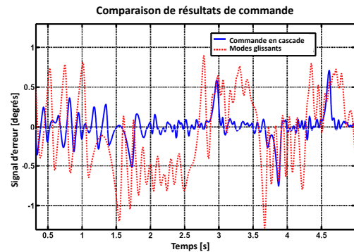
Fig. 9. Test de suivi avec un signal sinusoïdal à fréquence variable (chirp) : comparaison entre la stratégie en cascade proposée et les modes glissants
