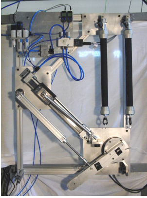
Fig. 1. Photo du banc expérimental.
