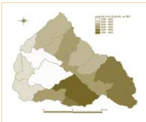
▼ Carte 2 – Flux d'azote simulés par sous-bassin en 2001 (kgN/km 2 ) (source : S. Berthelot).
