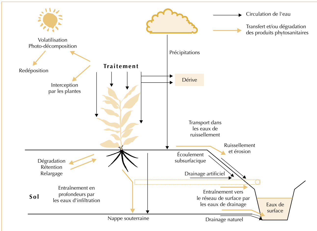
▲ Figure 3 – Schéma de collecte des flux d'eau et de produits phytosanitaires à la parcelle.
