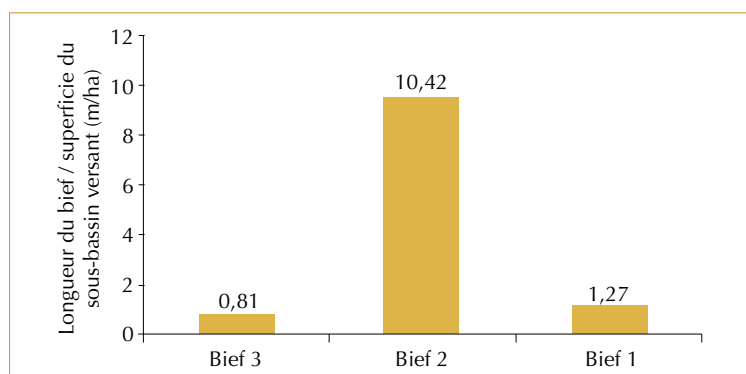
▲ Figure 4 – Rapports des longueurs de bief aux superficies des sous-bassins versants drainés pour les biefs identifiés.
