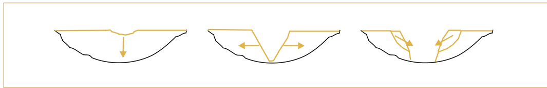
▲ Figure 7 – Évolution type d'une brèche par surverse. Vue en coupe rive/rive. La brèche s'approfondit puis s'élargit par érosion latérale ou par glissement des talus.
