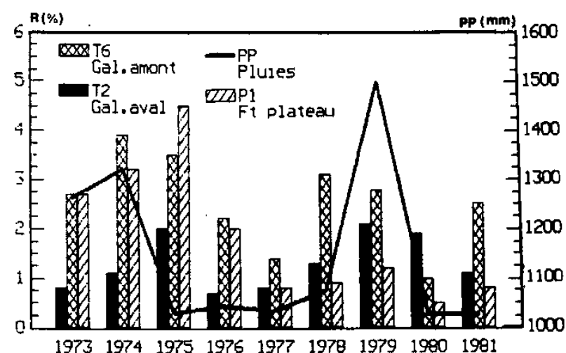
Fig. 3. — Précipitations et accroissements en surface terrière de trois peuplements forestiers au cours de 9 années successives à Lamto [gal. = forêt galerie (gallery forest); Ft. plateau = forêt de plateau ("plateau" forest)].
