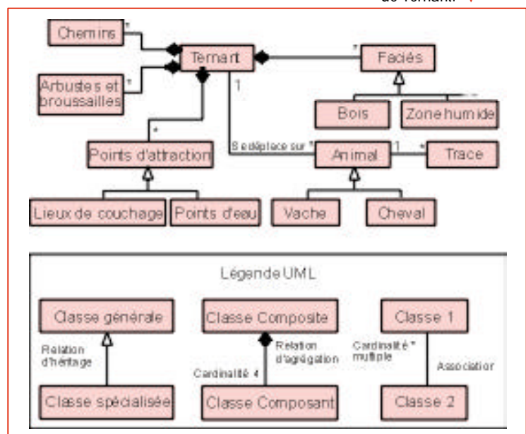
Figure 1. - Diagramme des classes UML du modèle conceptuel de Ternant. ▼
