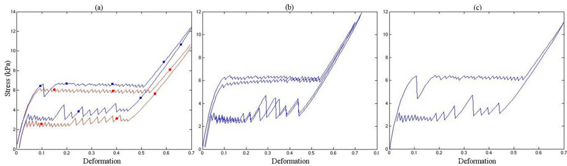
FIG. 6 (a) Courbes de réponse pour un système de 30 éléments : (a) deux essais à différente vitesse de chargement 5 mm/min (marqueurs ronds) et 100 mm/min (marqueurs carrés). (b) essai en compression cyclique sur échantillons vierges (b) et après une phase de repos de 72 heures (c).
