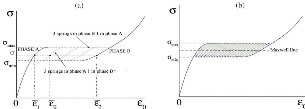
FIG. 5 Courbe de réponse d'une chaîne de 4 ressorts (a) et de 20 ressorts (b)
