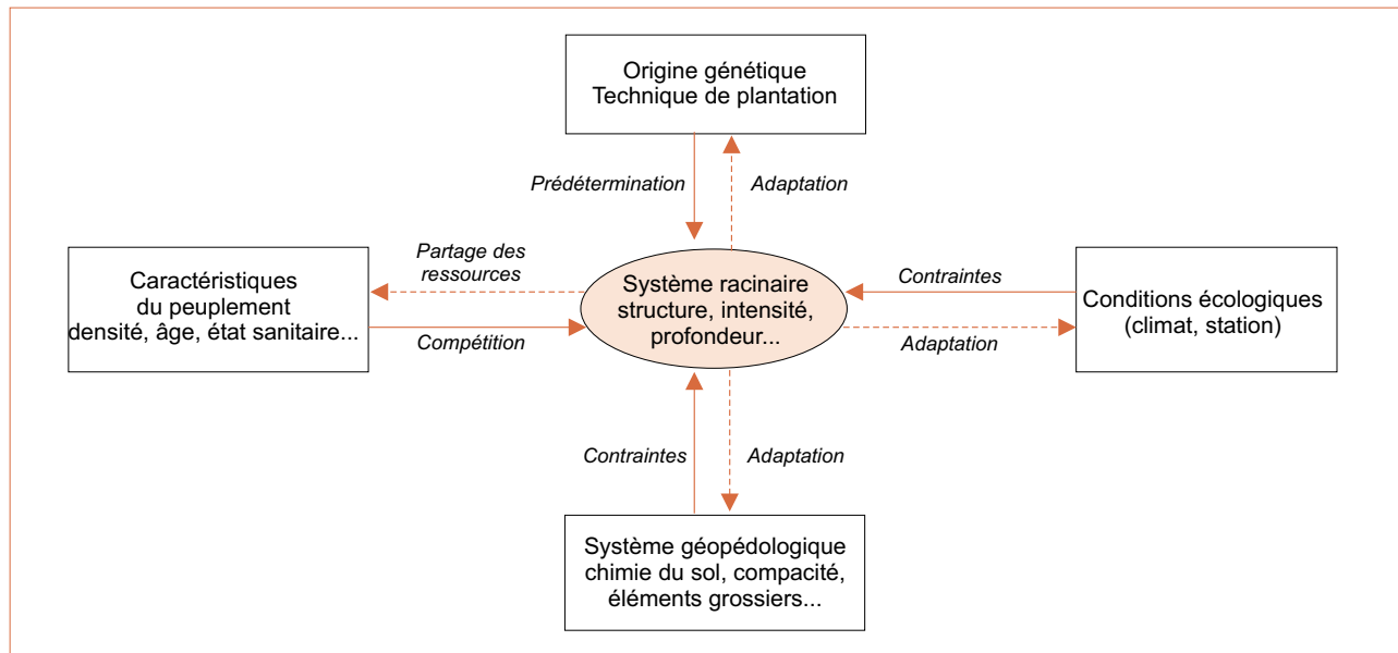
▲ Figure 1. – Les facteurs influant sur la morphologie et la structure du système racinaire.
