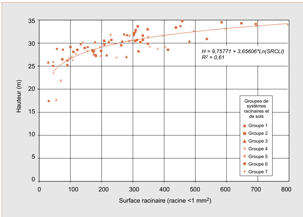
◀ Figure 8. – Relation entre la surface racinaire des racines fines et la hauteur dominante du Douglas à 35 ans.
