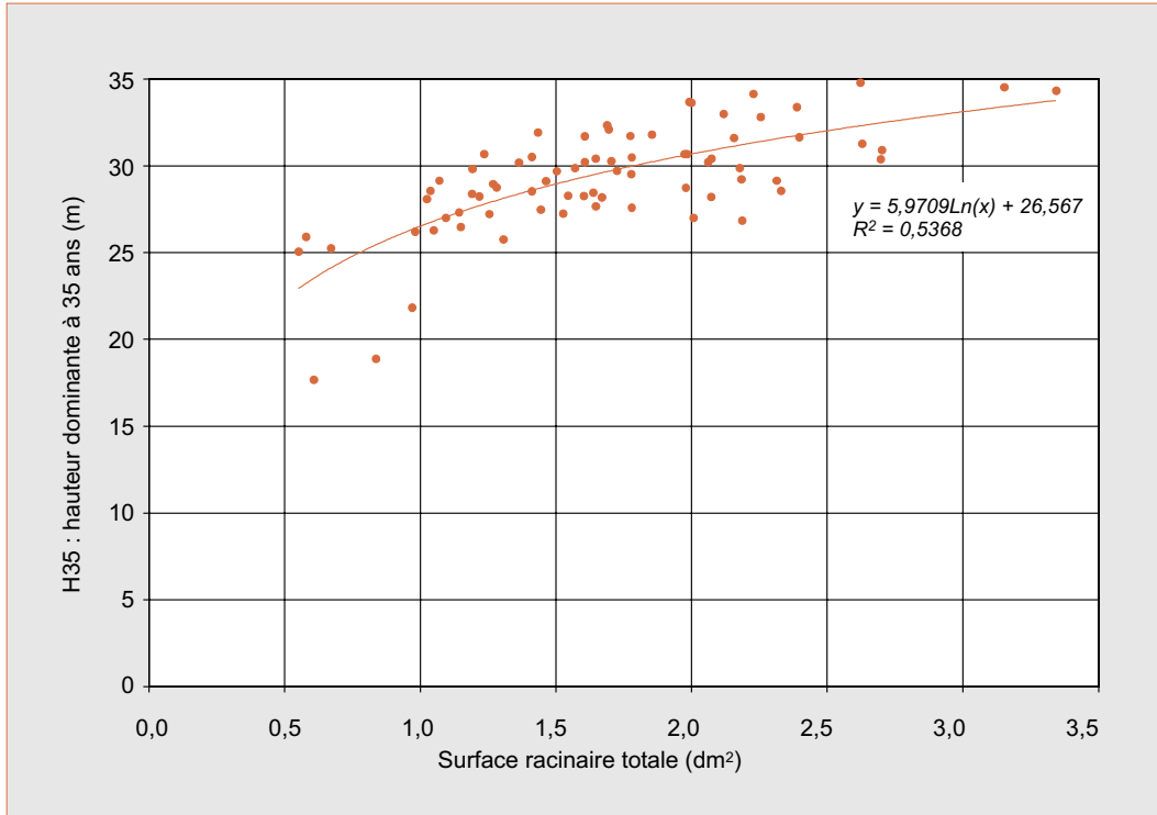
◀ Figure 7. – Relation entre la surface racinaire totale sur fosse et la hauteur dominante du Douglas à 35 ans.
