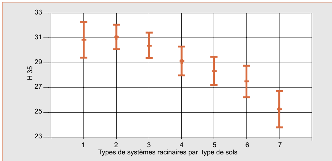
Figure 5. – Relation entre groupes systèmes racinaires par type de sols et hauteur dominante du Douglas à 35 ans.
