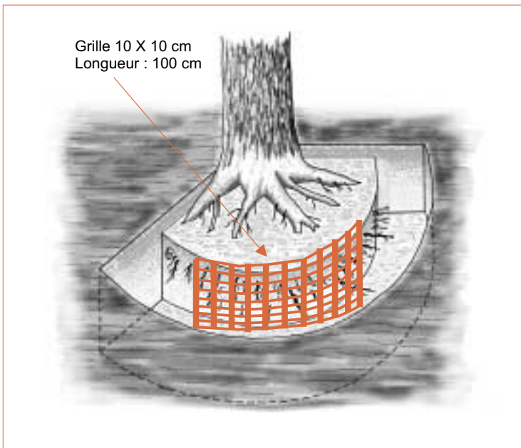
▲ Figure 3. – Méthode pour l'observation des sols et des systèmes racinaires.
