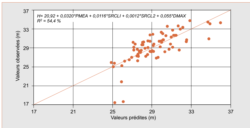
Figure 6. – Régression linéaire multiple entre variables racinaires et hauteur du Douglas (H35).
