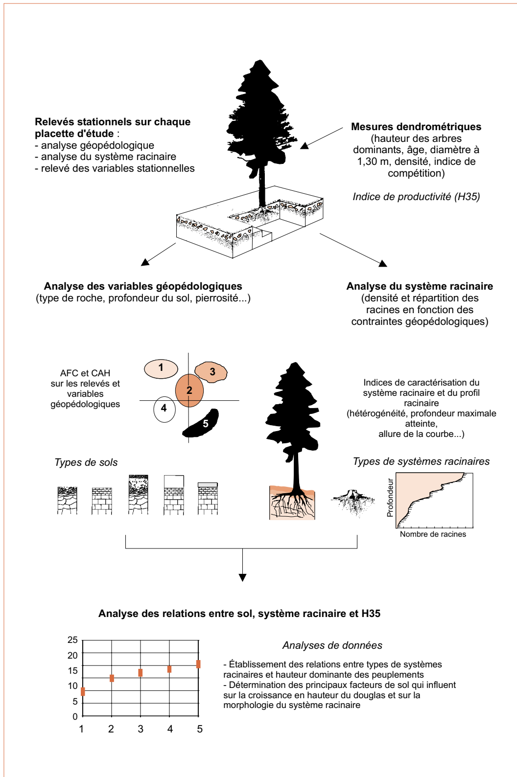
Figure 2. – Démarche de l'étude des sols et des systèmes racinaires.
