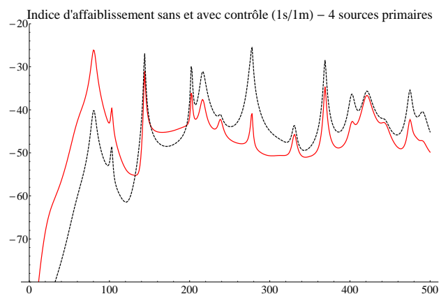
FIG. 3: Pertes par insertion de la plaque, en fonction de la fréquence. Rouge : sans contrôle ; Noire pointillée : avec contrôle par une source et un microphone.
