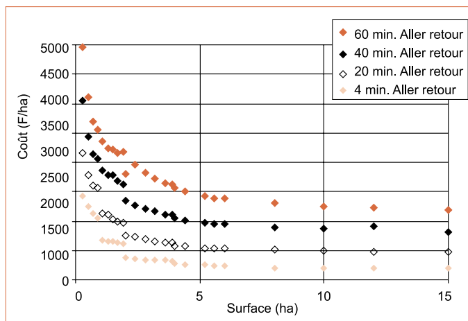
Figure 4. – Coûts de chantier par hectare en fonction de la surface et de la distance des chantiers d'ensilage. Cas d'une ensilieuse à 6 rangs (données modélisées). ▼
