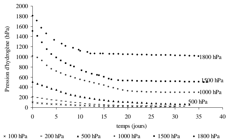
Figure 2. Variations de la pression d'hydrogène en fonction du temps pour différentes pressions initiales d'hydrogène (manométrie)
