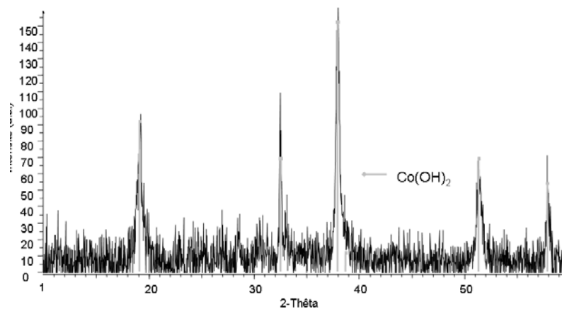
Figure 1. Diffractogramme de l'hydroxosulfure de cobalt initial
