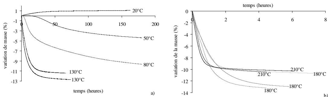
Figure 4. Effet de la température sur l'interaction H_2 -CoSOH à 20, 50, 80 et 130^\circ C (a) et 180 et 210^\circ C (b)
