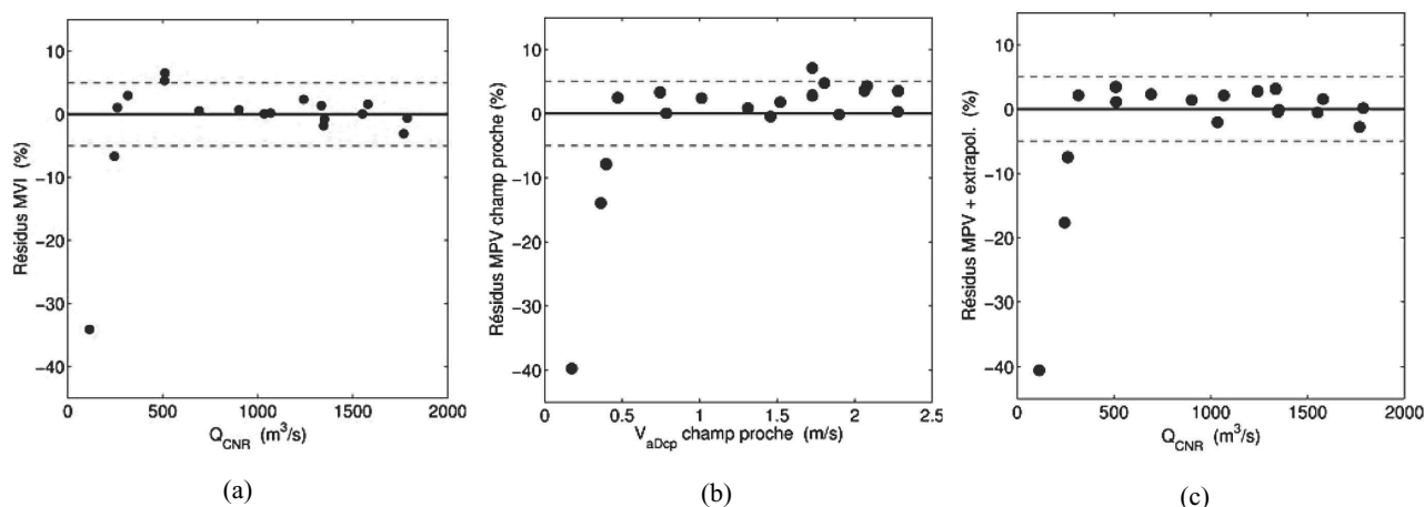
Fig. 6 – Résidus en débits/vitesses obtenus pour les différentes méthodes, par rapport aux valeurs jaugées : a) débits MVI ; b) vitesses moyennes MPV sur la sous-section scrutée correctement (profil log-constant) ; c) débits MPV (profil log-constant, avec extrapolation des vitesses à Froude constant en champ lointain).
