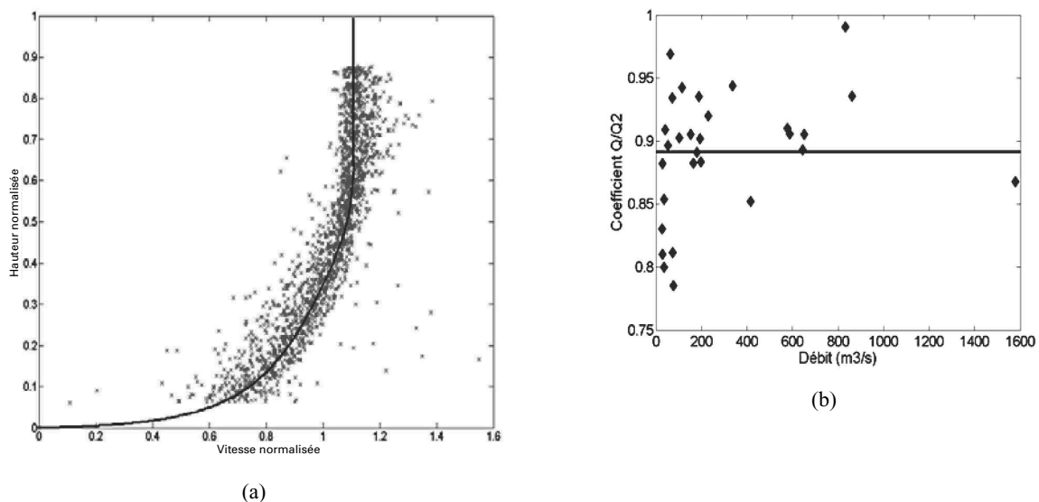
Figure 5 – (a) Profils adimensionnels de vitesse aDcp post-traités (points bleus) et profil log-constant calé (trait noir) ; (b) Rapport Q/Q_2 pour 29 jaugeages CNR au moulinet à Sauze.
