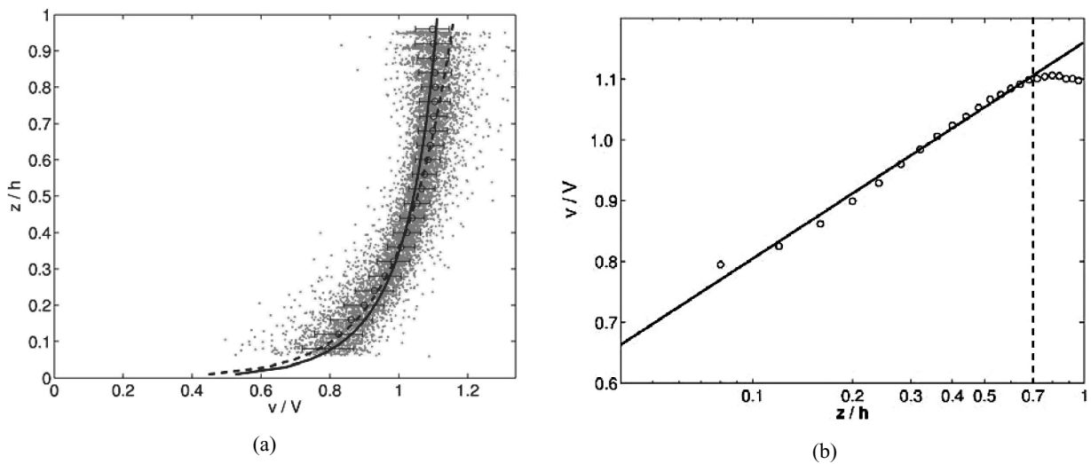
Fig. 4 – a) Profils adimensionnels de vitesse aDcp post-traités : nuage de points des 414 profils, profil moyen et écart-type expérimental (cercles), profil log calé (pointillés), profil de Van Rijn calé (ligne épaisse) ; b) Profil adimensionnel moyen (cercles) et calage logarithmique valable jusqu'à z/h = 0,7 .
