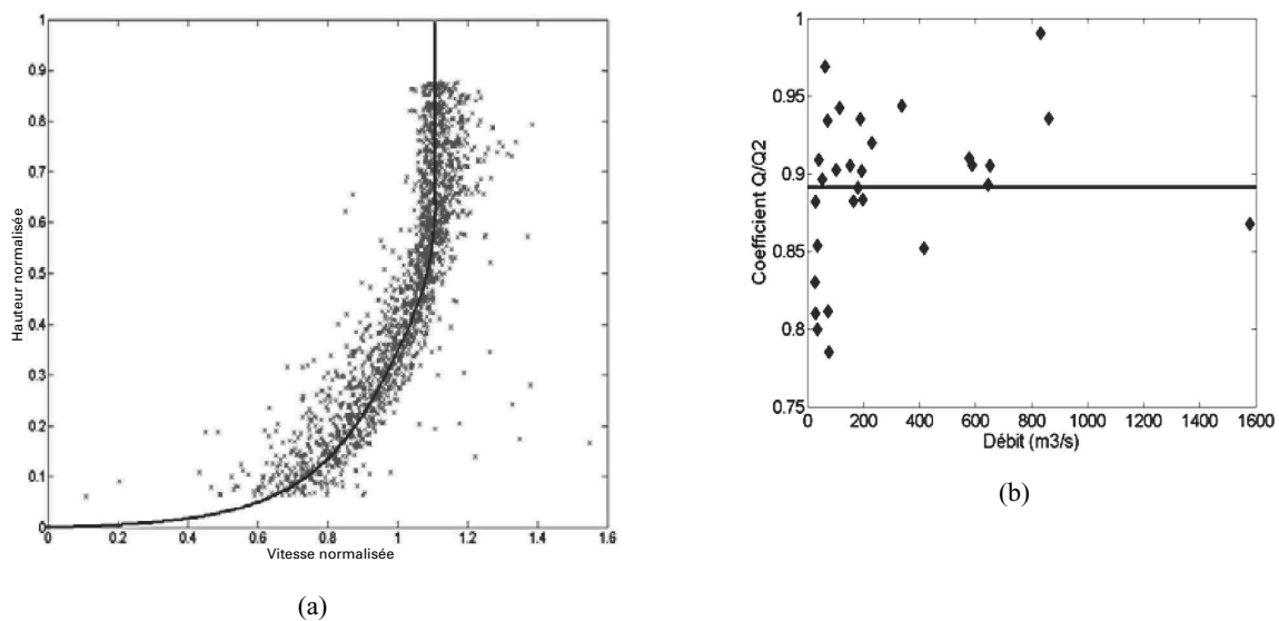
Figure 5 – (a) Profils adimensionnels de vitesse aDcp post-traités (points bleus) et profil log-constant calé (trait noir) ; (b) Rapport Q/Q_2 pour 29 jaugeages CNR au moulinet à Sauze.
