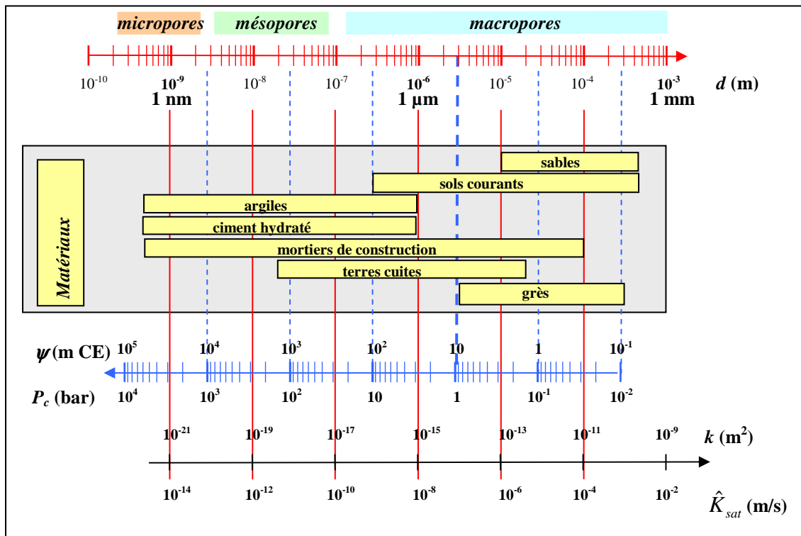
Fig. 7.14 Distribution pométrique de quelques matériaux, étalement correspondant de leur caractéristique capillaire (eau à 20°C) et évaluation de la perméabilité intrinsèque.
