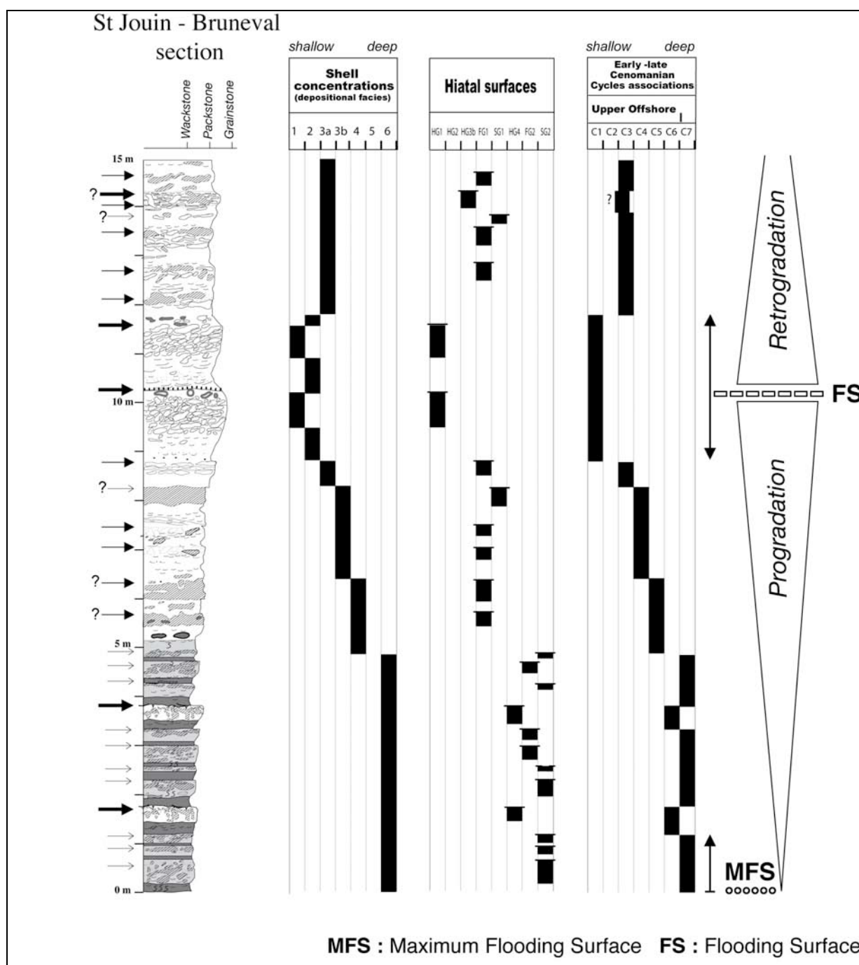
Figure 13: Exemple d'utilisation du modèle de faciès de la Craie cénomaniens sur la coupe de St Jouin-Bruneval
