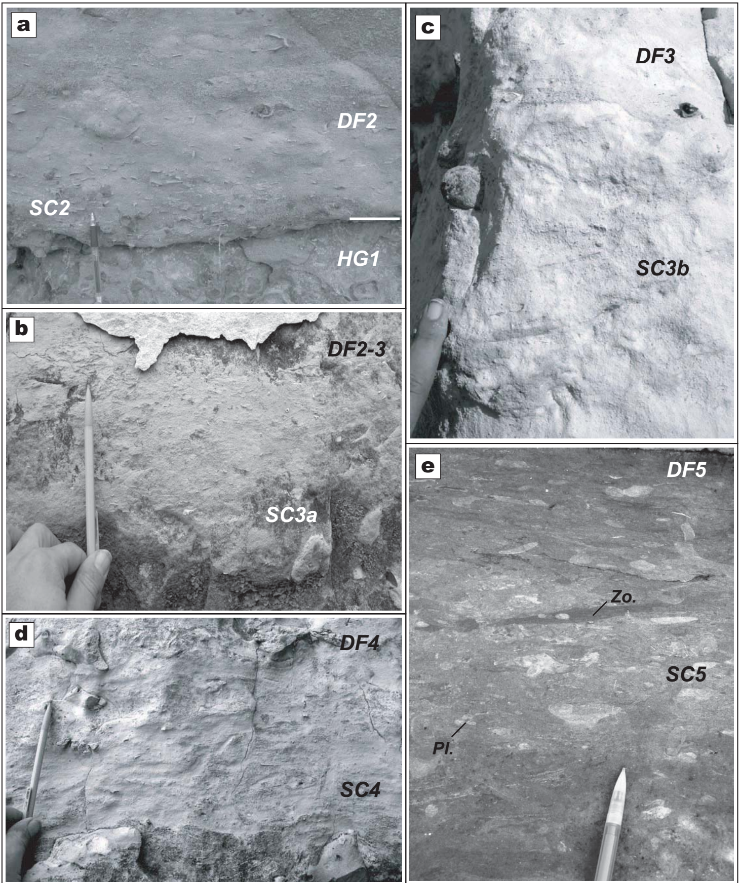
Planche 1: Principaux types de faciès en dépôt et concentrations de bioclastes associées.
