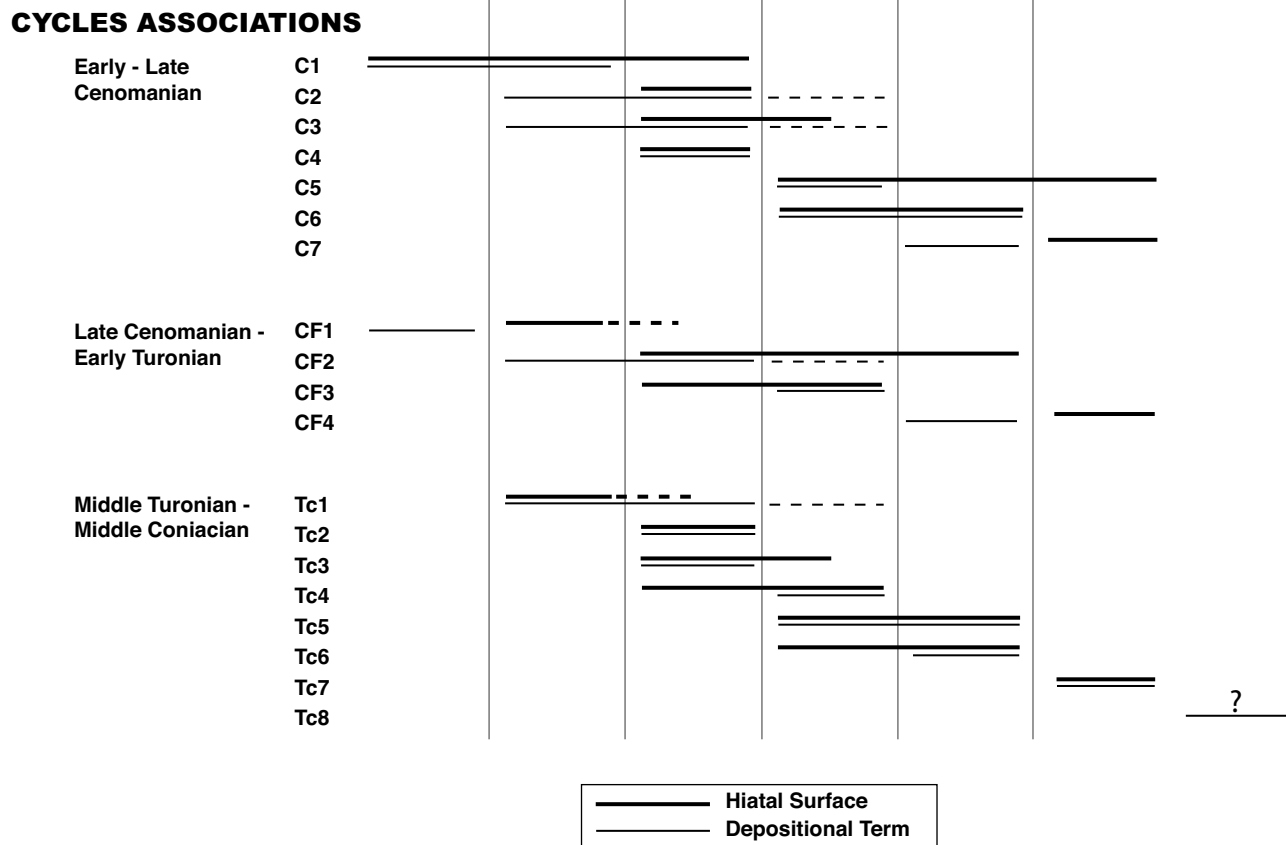
Figure 10: Distribution le long d'un transect proximal-distal des concentrations de bioclastes, des termes en dépôt et des surfaces d'arrêt de sédimentation (a), et utilisation des différents termes en dépôt et surfaces d'arrêt de sédimentation pour positionner les cycles des trois modèles de faciès le long d'un transect proximal-distal (b).
