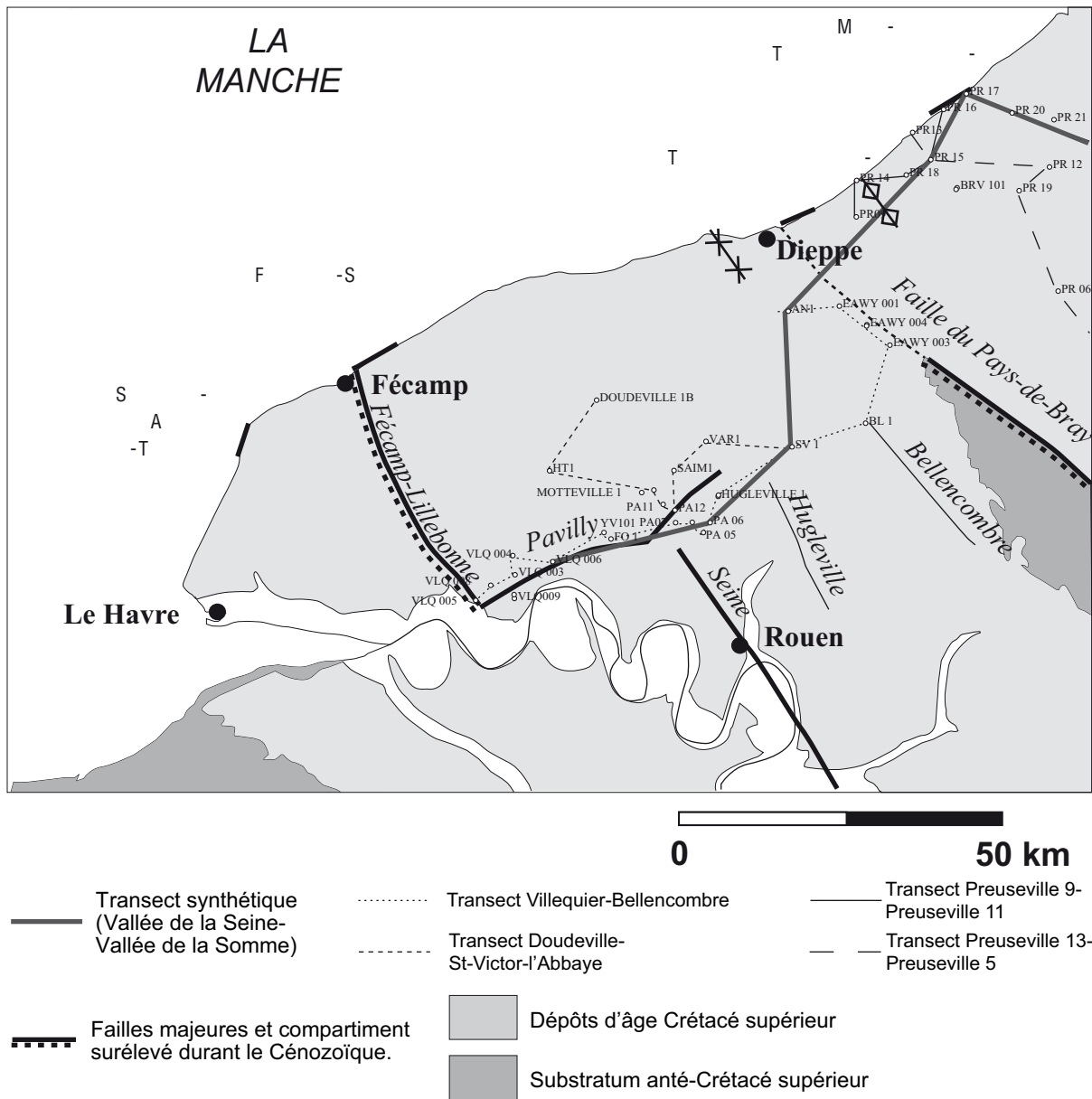
Figure 24: Carte géologique simplifiée de Haute-Normandie, position des différents puits diagramphés et transects réalisés.
