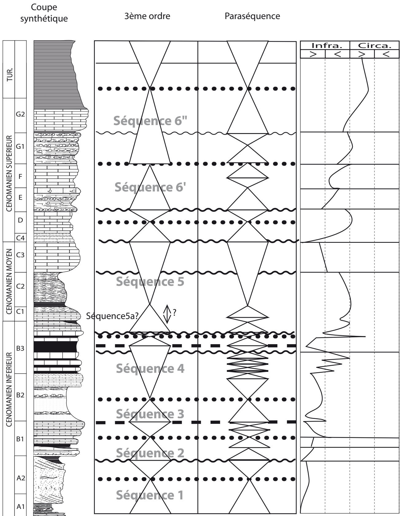
Figure 48 : Coupe synthétique, variations de plaéobathymétrie et proposition de modifications du découpage séquentiel, d'après Videt (2003), modifié.
