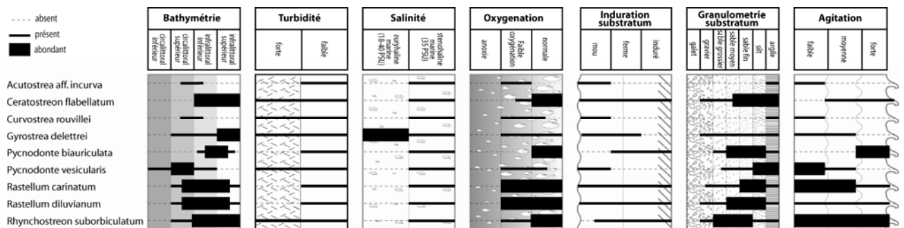
Figure 12 : Synthèse de distribution des principales huîtres cénomaniennes rencontrées en charentes en fonction de sept paramètres abiotiques (modifié, d'après Videt & Néraudeau 2007).
