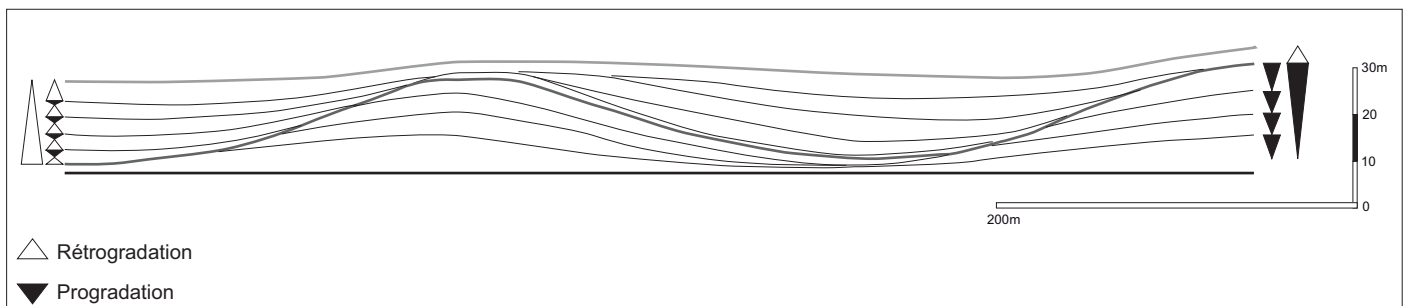
Figure 31: Géométrie élémentaire des corps sédimentaires et évolution de ces géométries en relation avec les variations du niveau marin.
