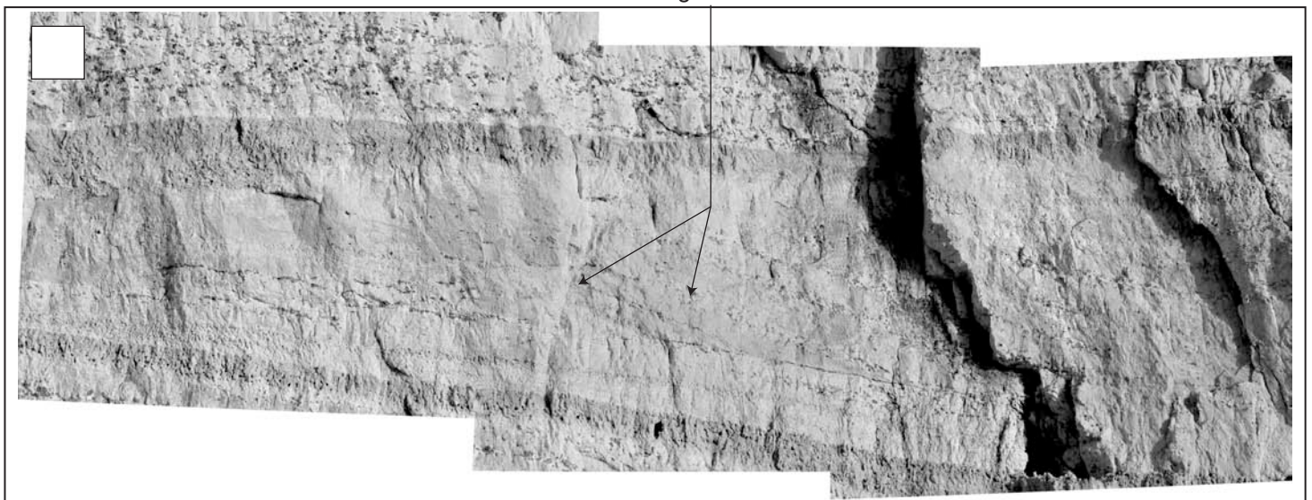
Mégarides 2D
