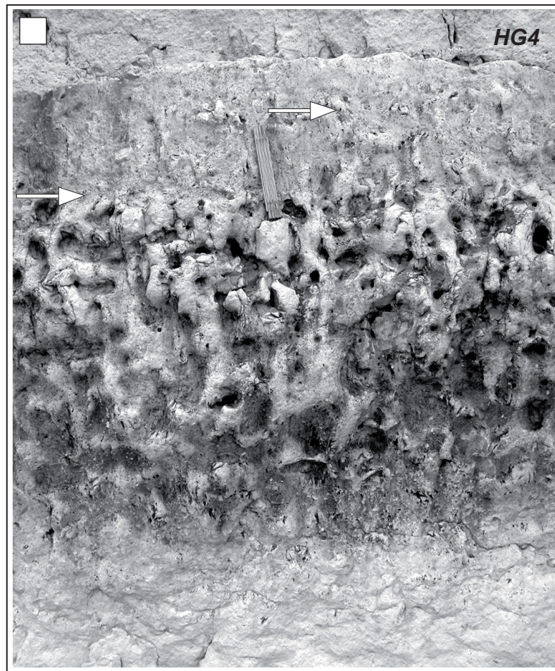
Planche 3: Hardgrounds 3 et 4. Les flèches blanches indiquent le sommet de la surface principale. a: Zoom sur un hardground HG 3a. Remarquer l'abondance de clastes et la granulométrie élevée. Cénomaniens supérieur, Coupe du Cap Fagnet. b: HG3b, remarquer la surface très plane de ces hardgrounds et les clastes au dessus de celle-ci. Coniacien inférieur, Coupe Penly-Dieppe. c: HG4, remarquer l'absence de troncature en sommet de ces hardgrounds, visible par des nodules branchus au dessus de la surface principale. Turonien supérieur, Coupe de Criel.
