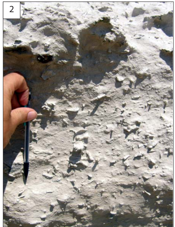
Planche 15 :Faciès de la coupe Les Monards-Pilou: 1: Faciès de la base de la coupedes Monards; 2: faciès de la base de la Coupe du Pilou., 3: Lumachelle à pycnodontes de la coupe du Pilou 4: faciès de la partie supérieure de l'unité CIV b, 5: Faciès de l'unité CV.
