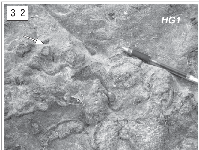
Planche 6: Faciès intermédiaires et proximaux du Cénomaniens (points 2 et 3 de la figure 14).
