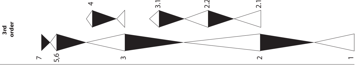
Figure 17: Mode d'empilement des cycles sédimentaires, variations de milieu de dépôt et découpage séquentiel de la Coupe St Jouin-Bruneval.
