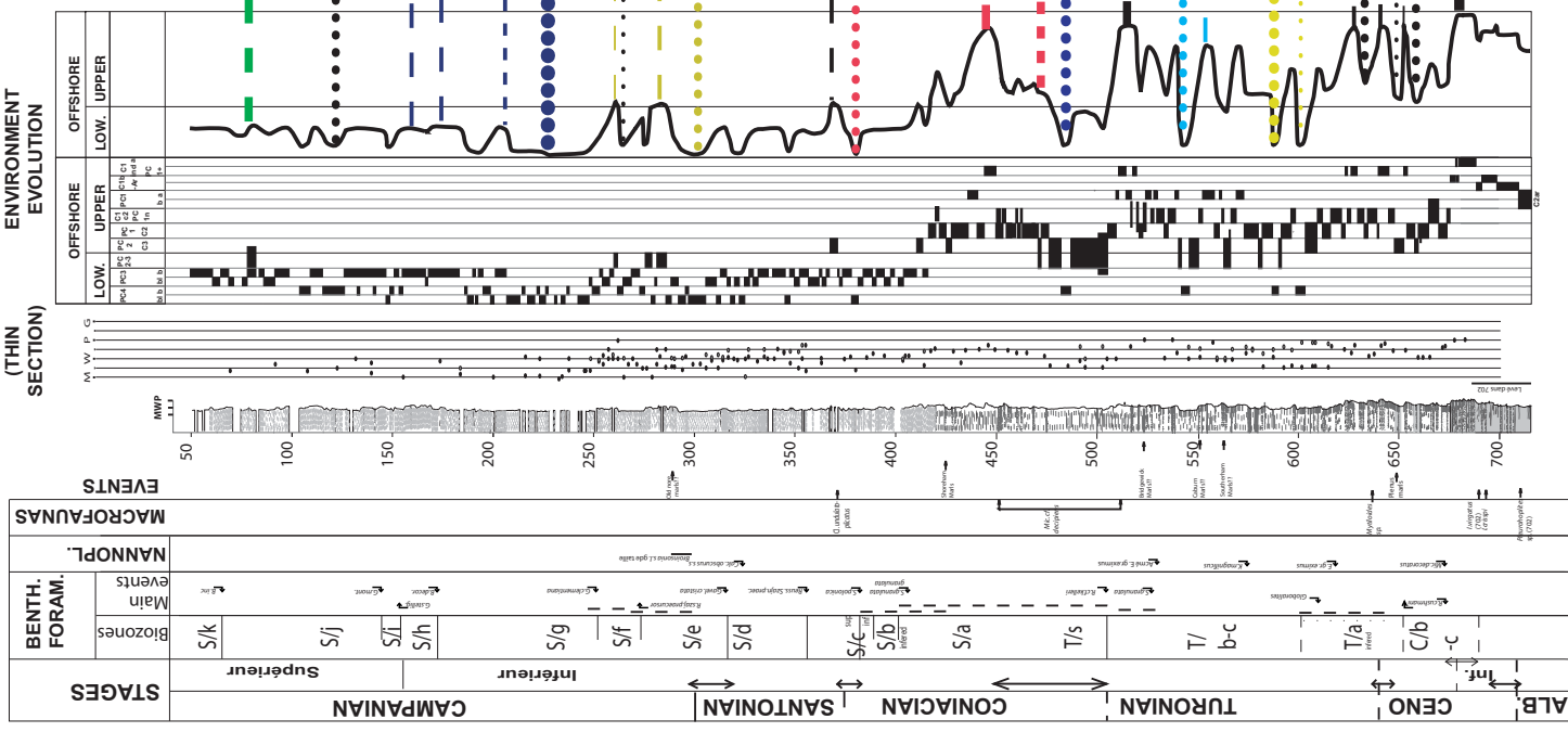
Figure 51 : Comparaison des coupes synthétiques du Bassin de Paris (forage Craie 700) et de la plate forme Nord Aquitaine composites de Craie 700 et de la plate forme nord aquitaine Coupe composite du forage Craie 700, variations d'environnement de dépôt et découpage séquentiel. Stratigraphie de Craie 700 d'après Robaszynski et al., 2005; Robaszynski et al., 2000; Janin (2000).
