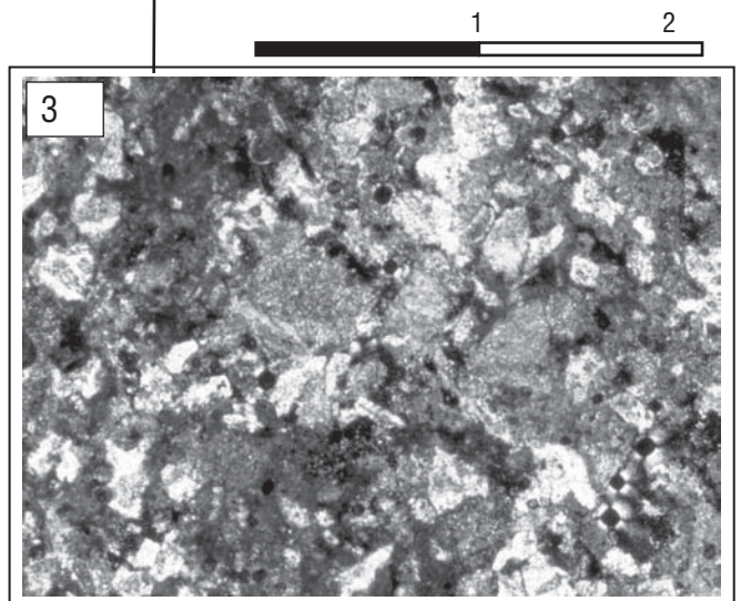
Planche 6: Faciès intermédiaires et proximaux du Cénomaniens (points 2 et 3 de la figure 14).
