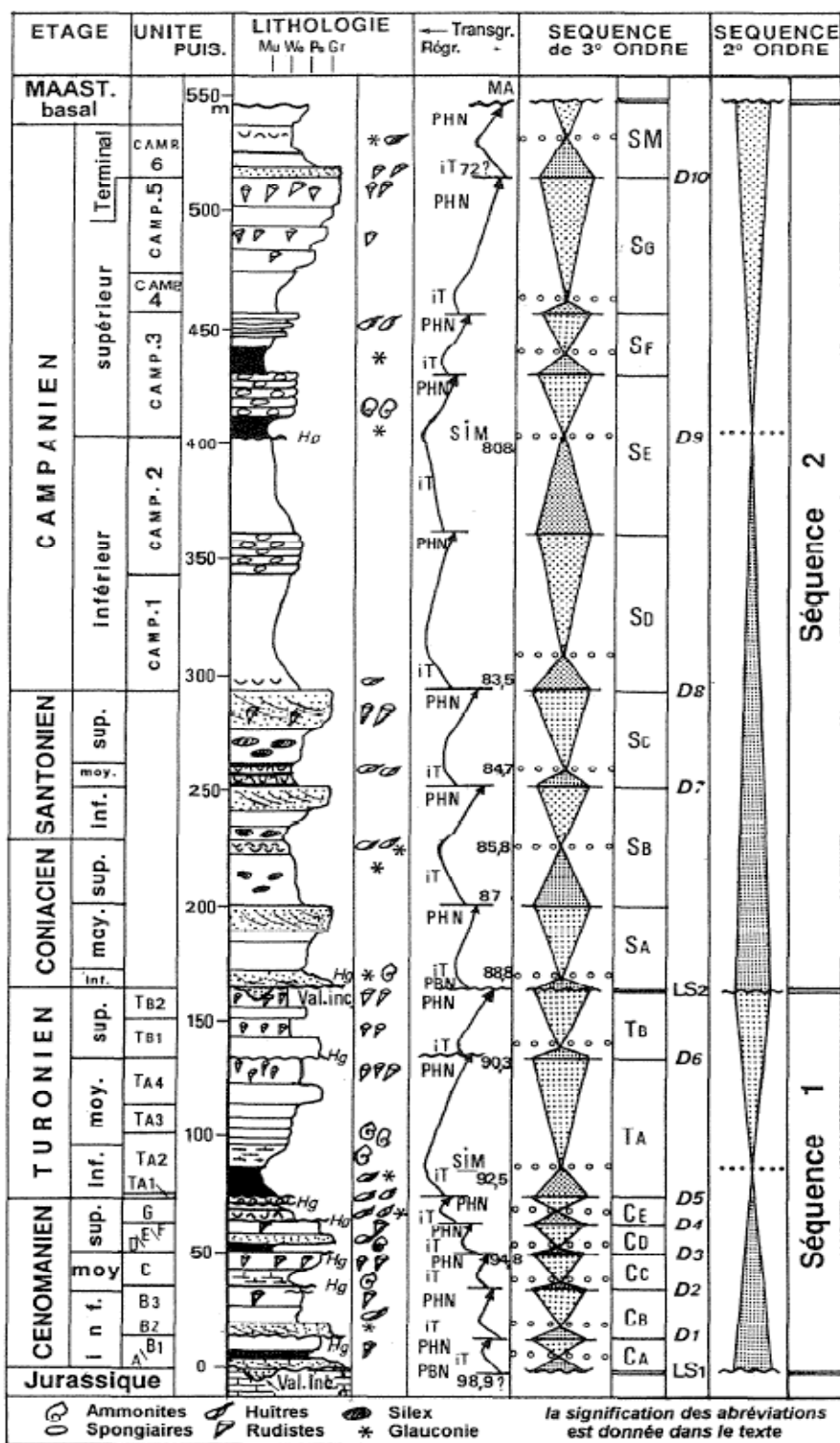
Figure 37 : Coupe synthétique et stratigraphie séquentielle de la plate-forme Nord Aquitaine, d'après Platel, 1996
