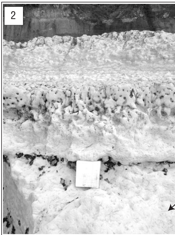
Planche 8: Faciès rencontrés en base de la formation de Senneville (hardgrounds Tilleul et niveaux immédiatement sus-jacents) position sur la figure 19.
