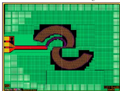
Figure 6 : Schématique de l'antenne double spirale avec dummies après cadence ®
